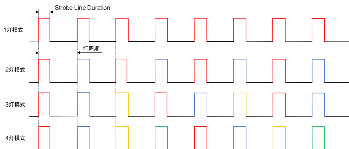
图10-37 IO 输出脉冲示意图
