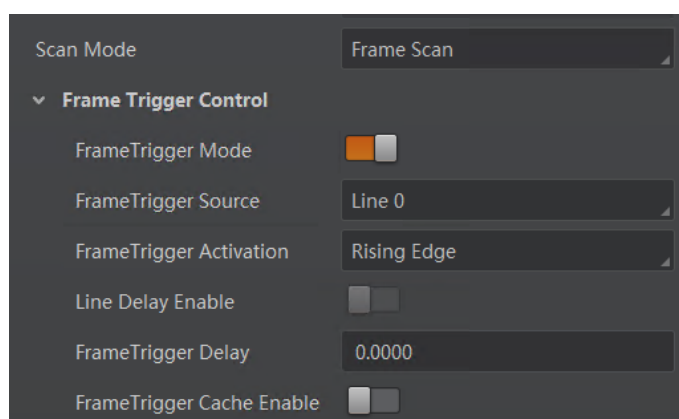
图8-14 帧触发响应方式
