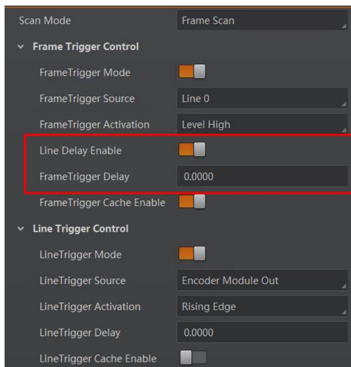
图8-25 延迟时间设置
