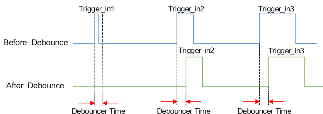
图8-23 触发防抖时序
