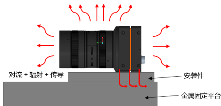
图4-10 安装件散热
