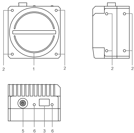
图4-6 第六种相机外观
