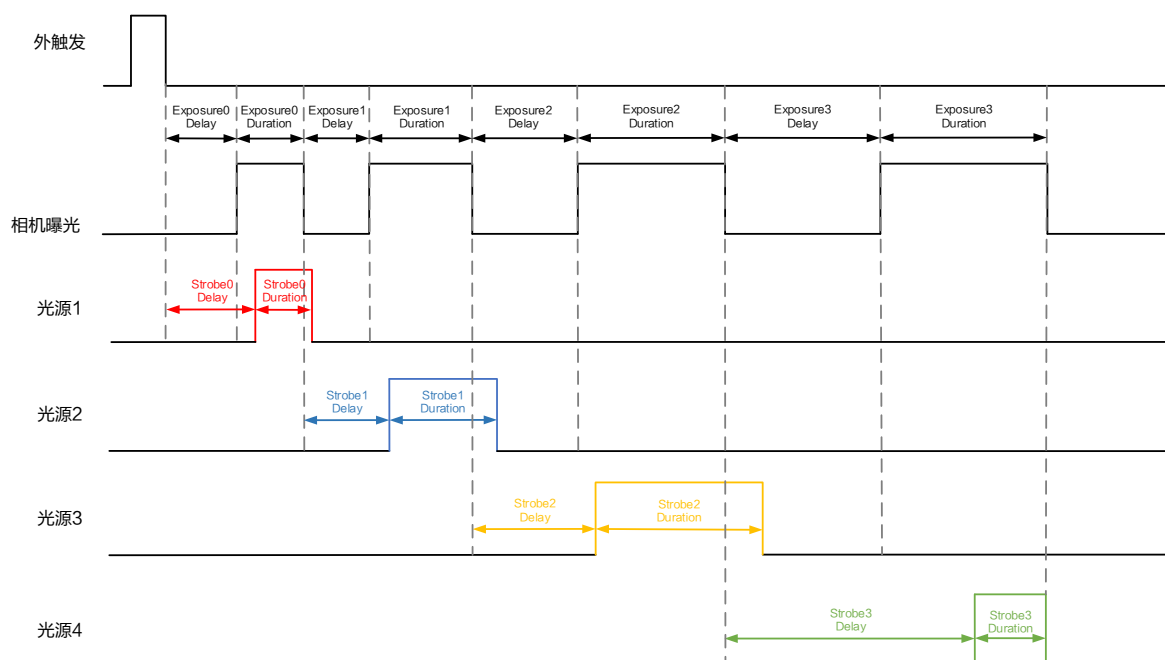
图10-41 4 灯模式触发示意图
