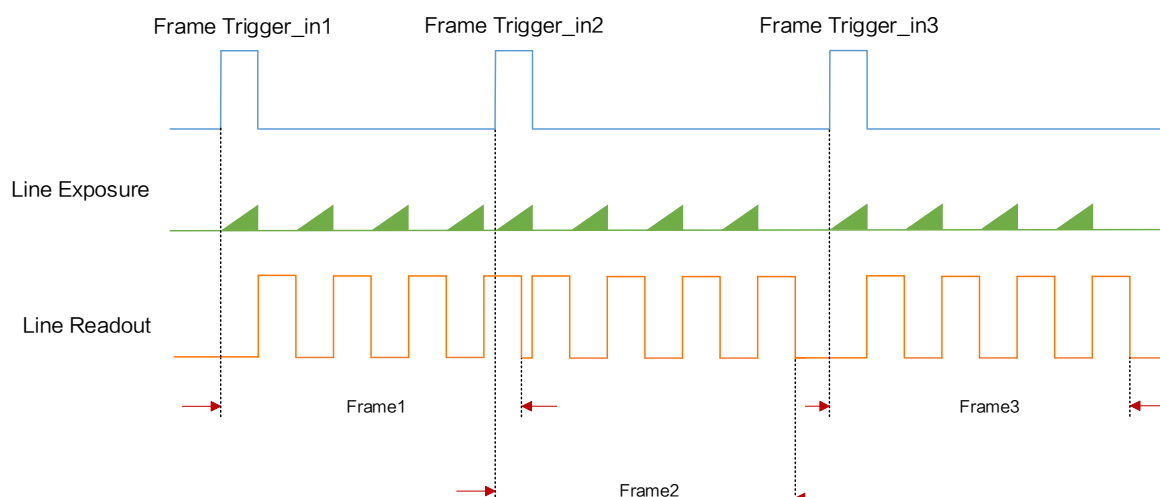
图8-19 第 2 帧正常处理时序
