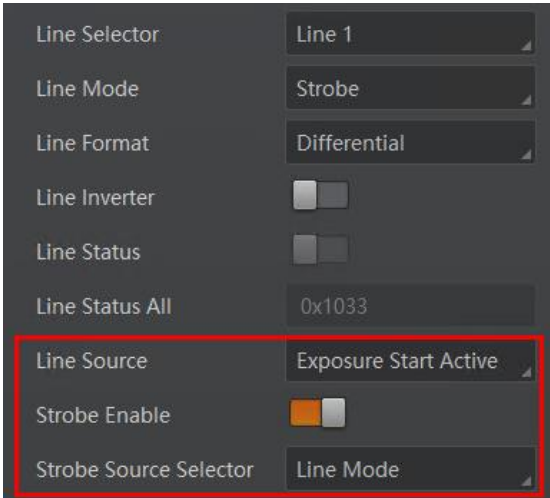
图8-29 Line Mode 模式
