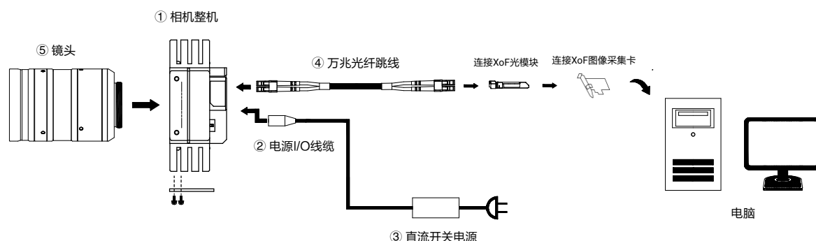
图6-1 整机连接
