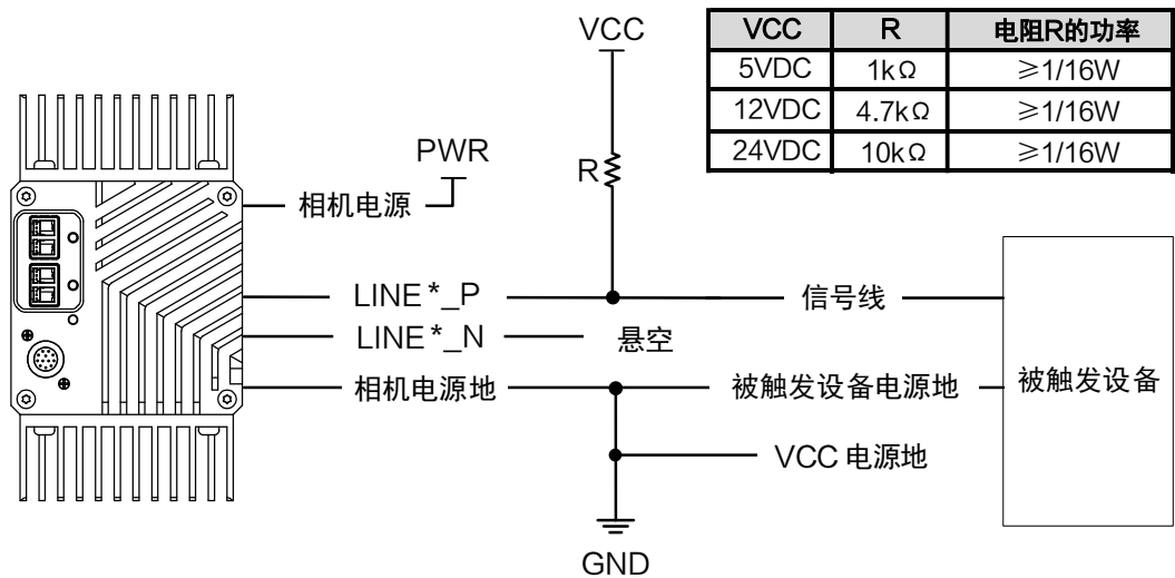
图7-9 单端输出接线（需上拉电阻）
