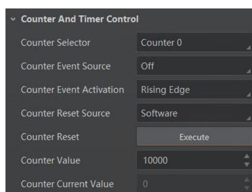
图8-30 计数器触发设置
