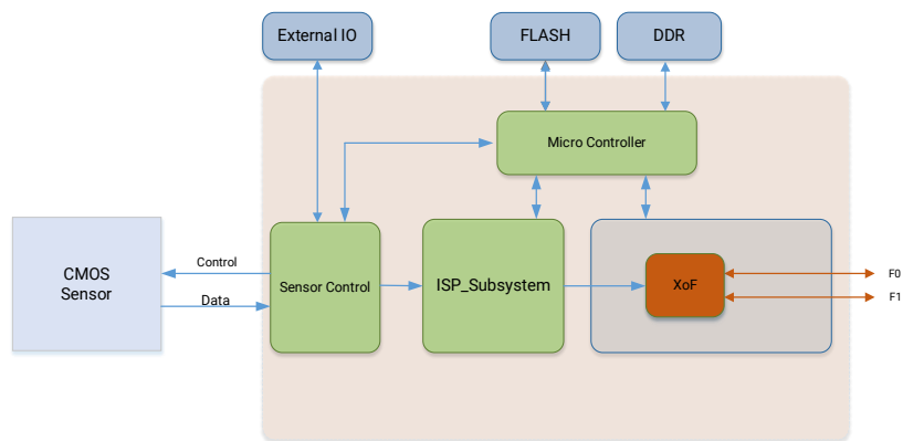
图3-1 工作原理
