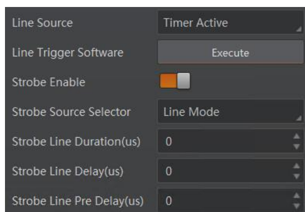
图8-31 Timer Active 相关参数
