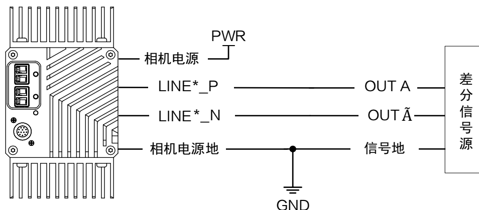
图7-3 差分输入接线
