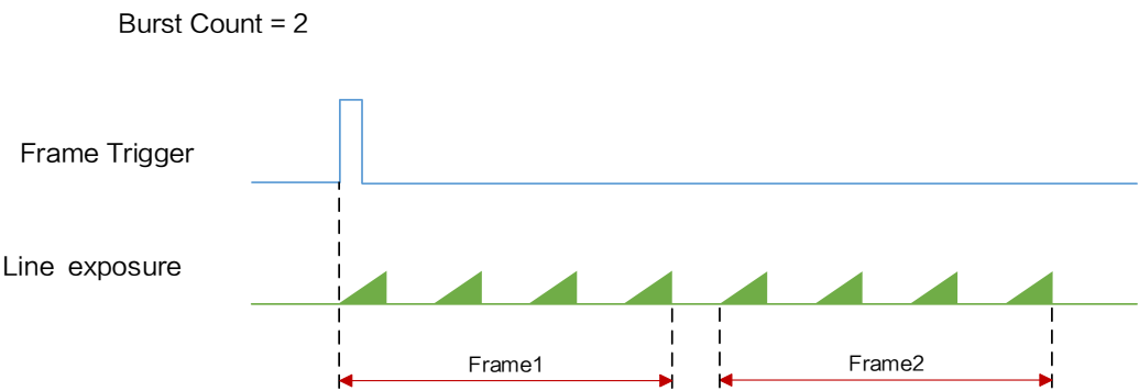
图8-13 触发出图数时序
