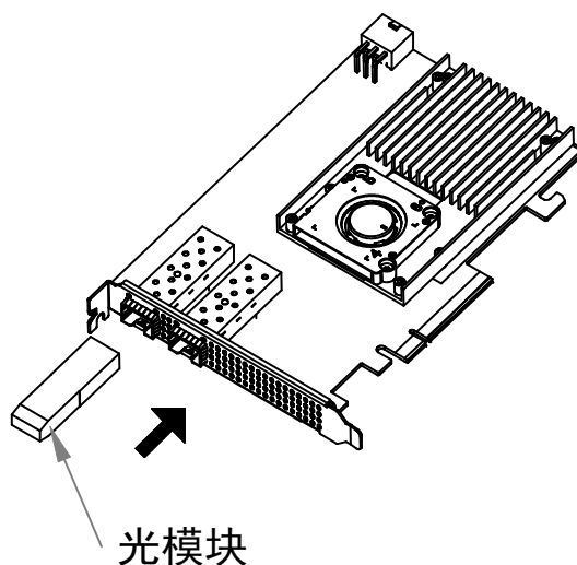
图6-2 将光模块插入采集卡
