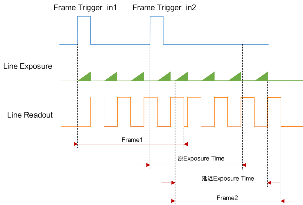
图8-20 第2帧曝光移动处理时序
