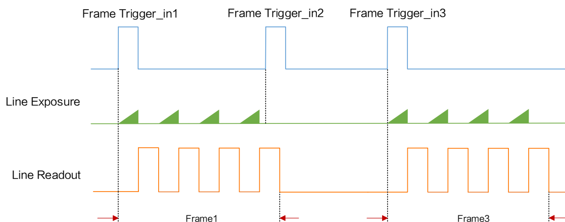
图8-18 第 2 帧被过滤时序
