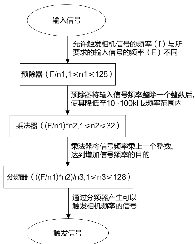
图8-8 频率转换流程图
