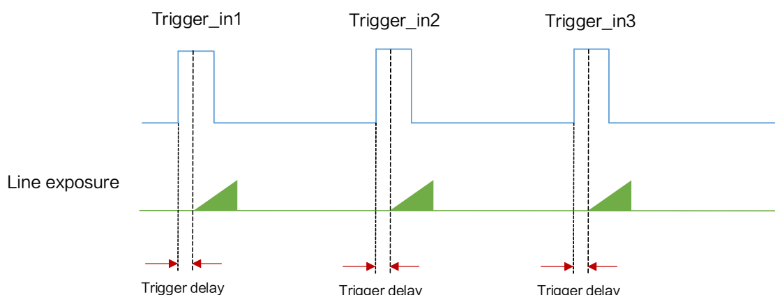
图8-24 信号延迟原理
