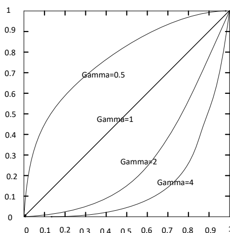
图10-19 Gamma 曲线图
