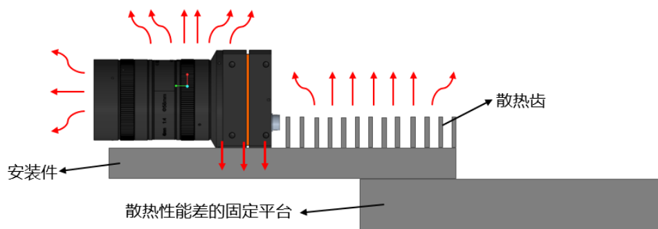
图4-13 增加散热齿的安装件
