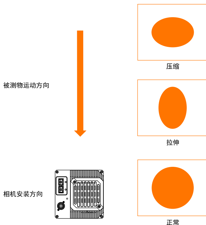
图9-2 行频调整效果
