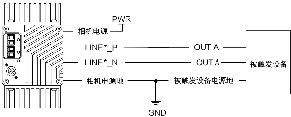
图7-8 差分输出接线
