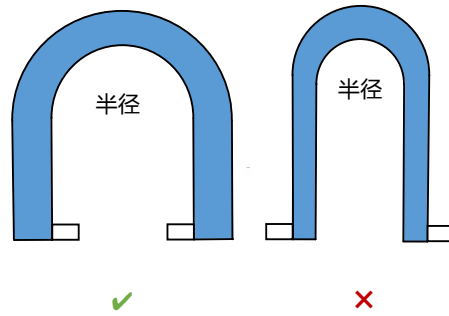
图5-5 足够的弯曲半径
