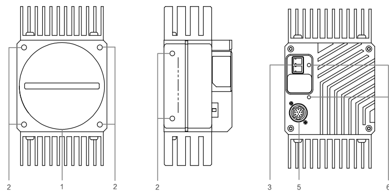
图4-2 第二种相机外观
