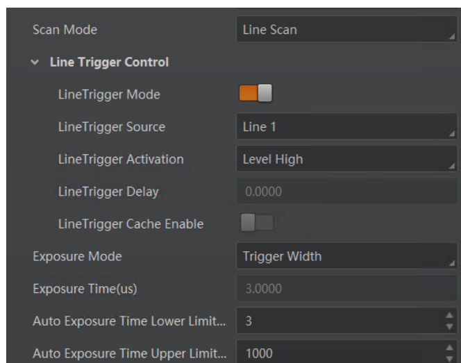
图8-16 行触发响应方式
