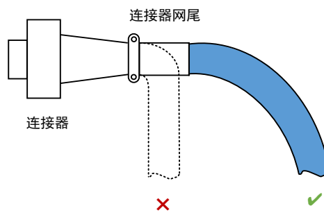
图5-6 装配连接器
