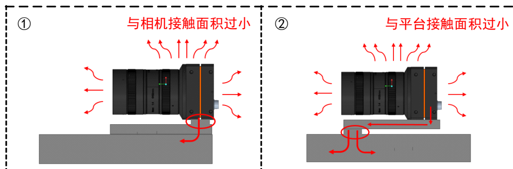
图4-12 安装件与相机、固定平台之间的接触面积
