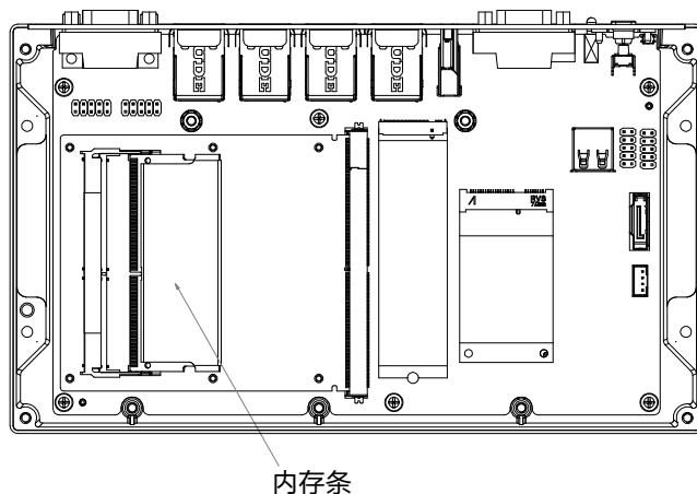
图4-2 内存条
