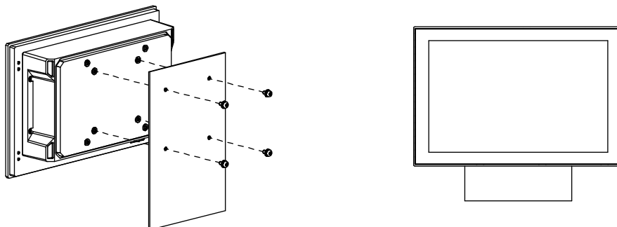
图3-4 壁挂式安装
