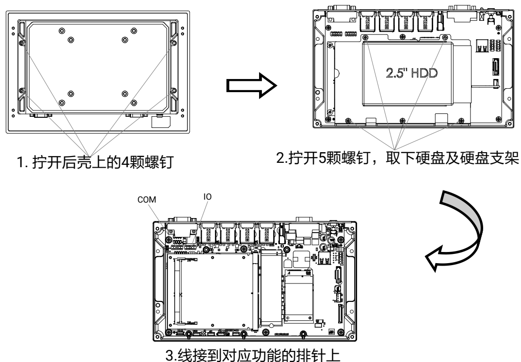
图4-12 IO/COM 功能切换操作
