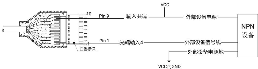
图4-15 输入接 NPN 设备（不使用上拉电阻）
