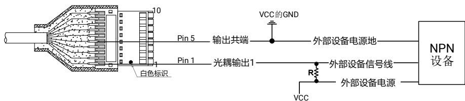
图4-11 输出接 NPN 设备（使用上拉电阻）
