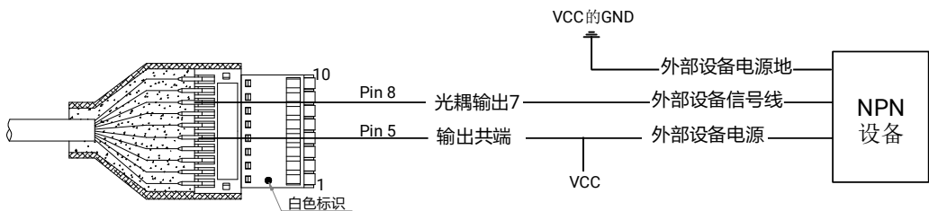
图4-18 输出接 NPN 设备（不使用上拉电阻）
