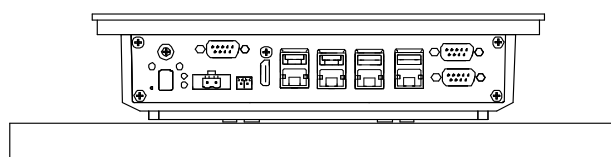
图3-1 台面放置
