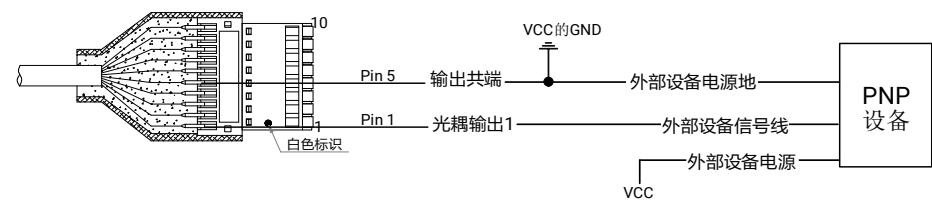
图4-9 输出接 PNP 设备
