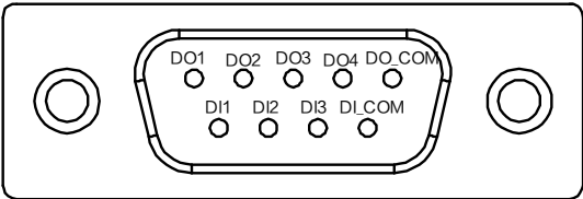
图4-5 IO 接口引脚
