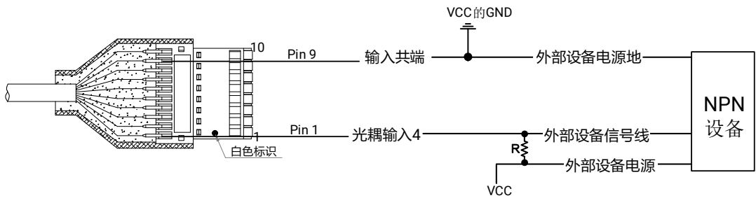
图4-16 输入接 NPN 设备（使用上拉电阻）
