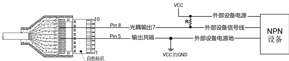
图4-19 输出接 NPN 设备（使用上拉电阻）
