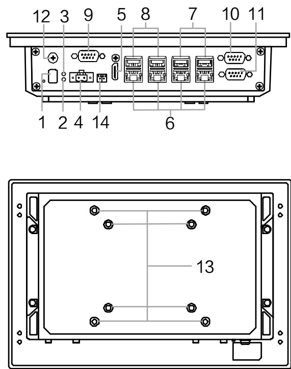
图2-1 设备外观
