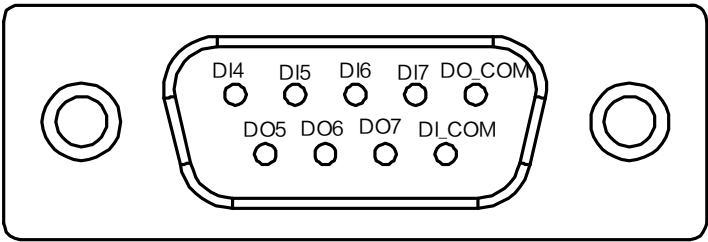
图4-13 IO 接口引脚
