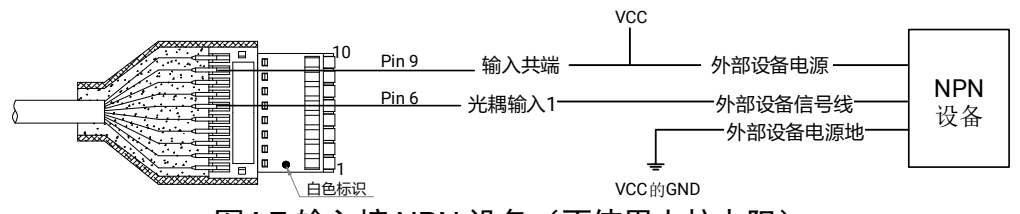
图4-7 输入接 NPN 设备（不使用上拉电阻）
