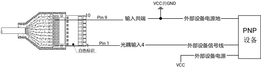
图4-14 输入接 PNP 型设备
