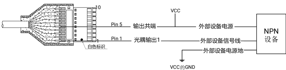
图4-10 输出接 NPN 设备（不使用上拉电阻）
