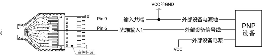
图4-6 输入接 PNP 型设备
