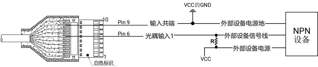
图4-8 输入接 NPN 设备（使用上拉电阻）
