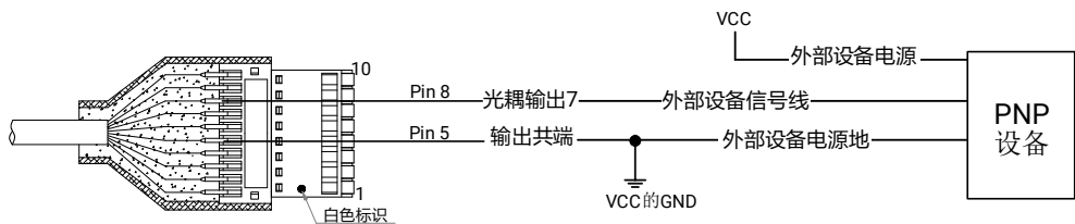
图4-17 输出接 PNP 设备
