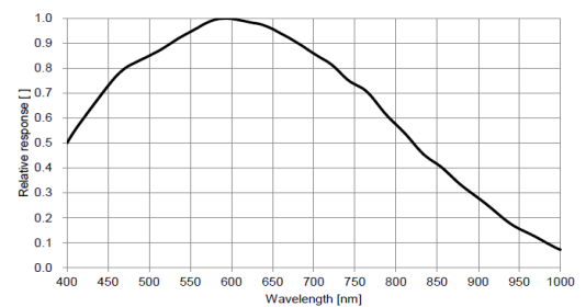
MV-CB016-10GM 量子效率
