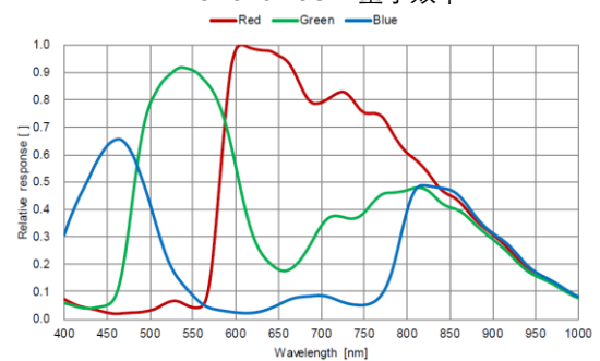
MV-CB016-10GC 量子效率
