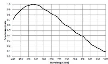
MV-CB060-10UM 量子效率
