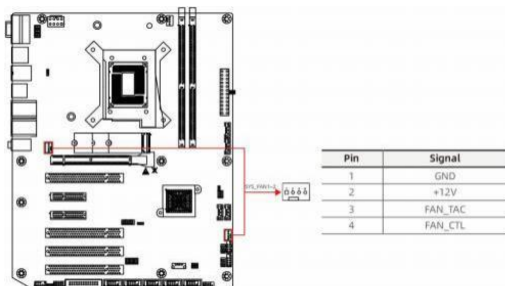
图 5-8 系统风扇 SYS_FAN 接口
