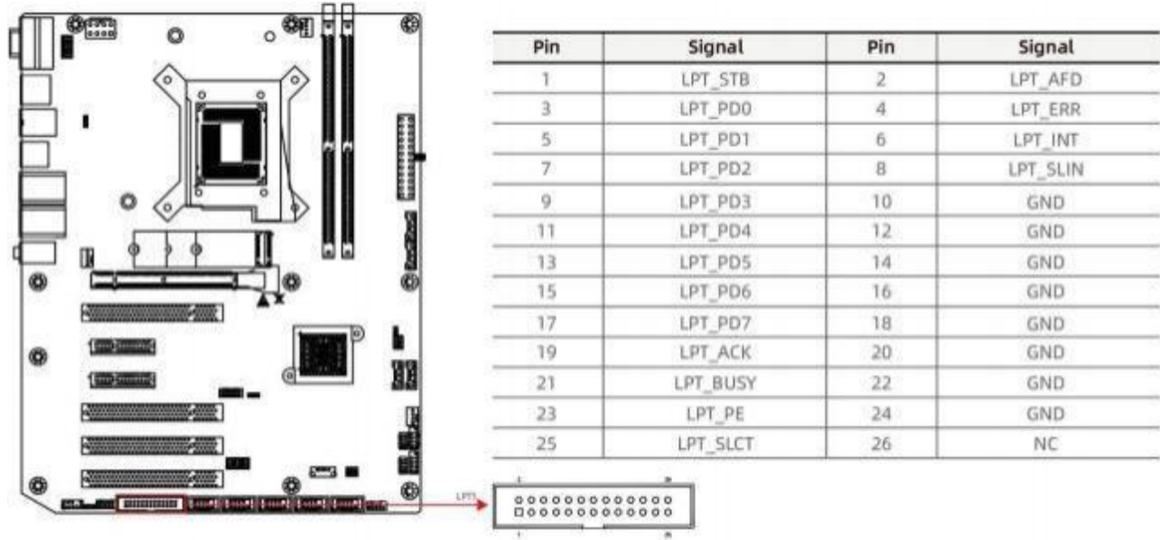
图 5-11 LPT1 接口
