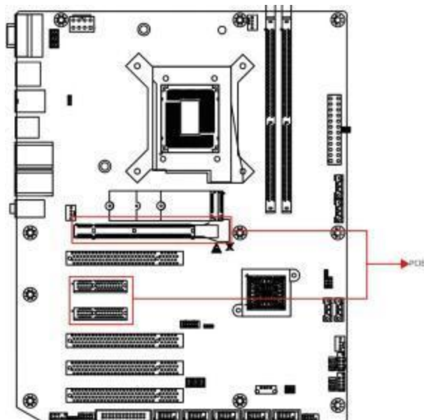
图 5-13 PCIe 接口
