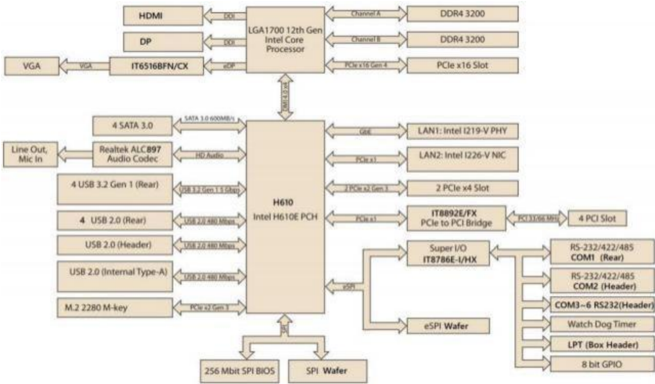
图 2-1 主板架构图
