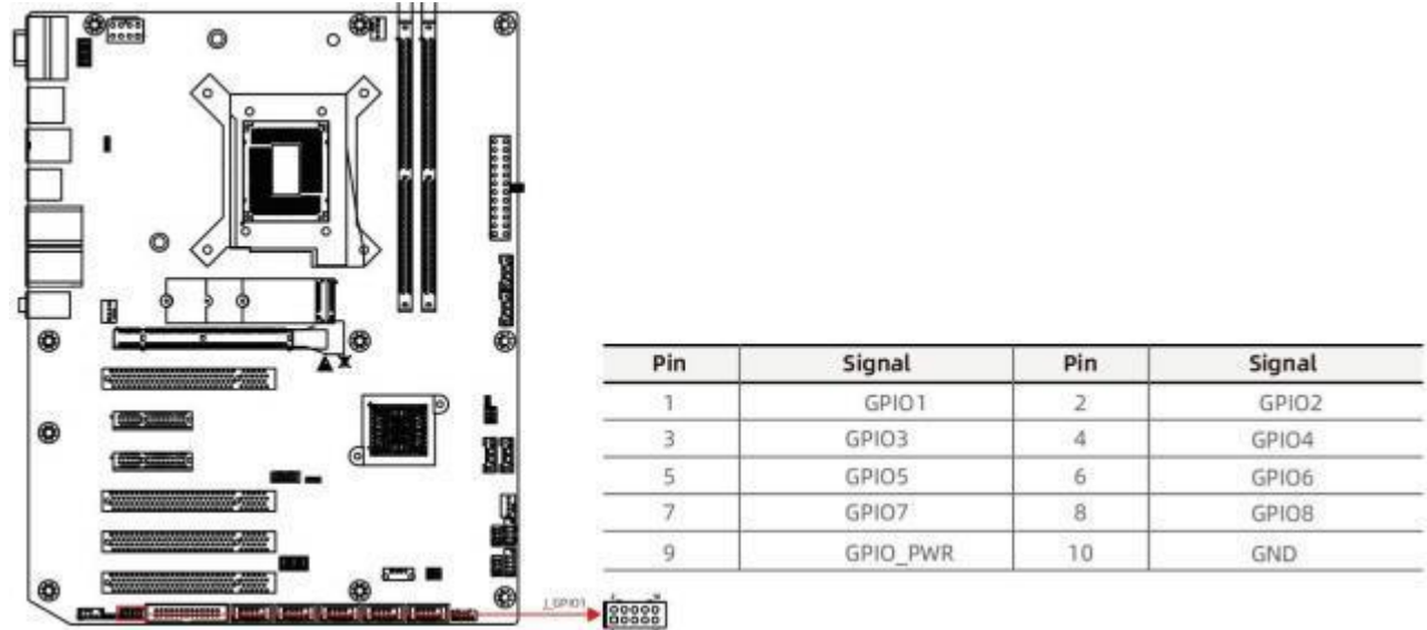
图 5-12 J_GPIO1 接口
