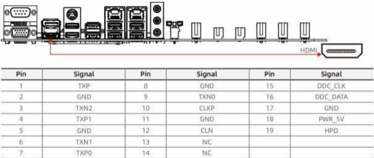
图 4-4 HDMI 接口
