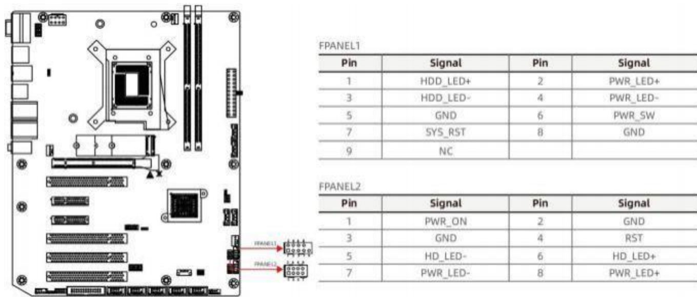
图 5-9 前置面板控制信号 FPANEL1/2 接口
