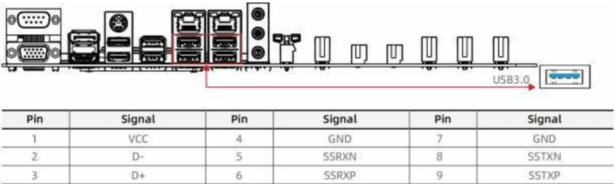
图 4-8 USB3.0 接口
