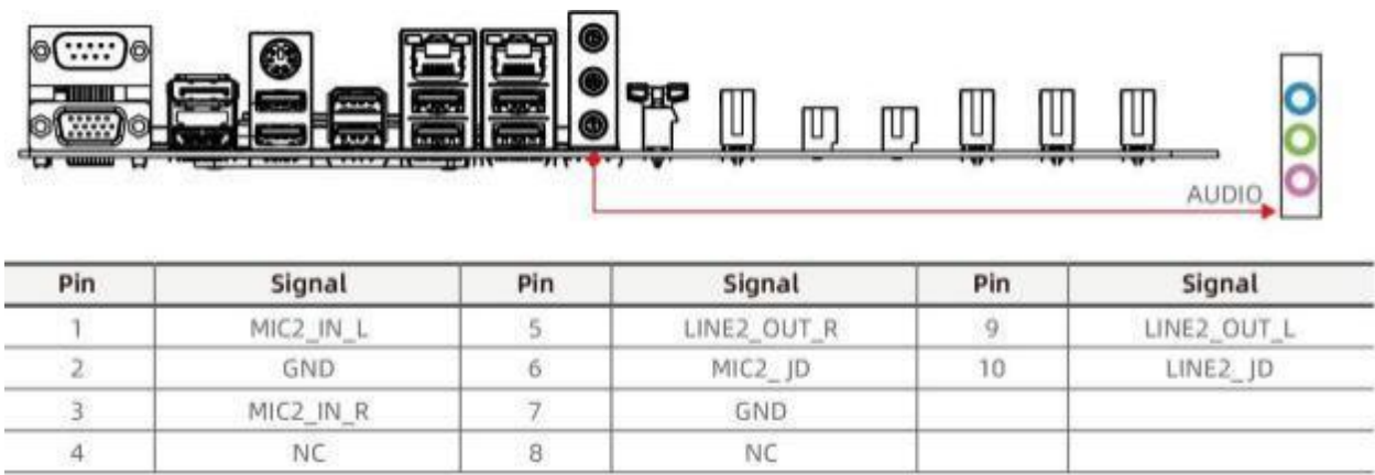
图 4-9 音频接口
