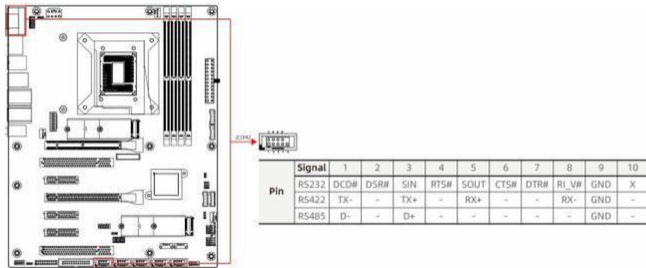
图 5-3 JCOM2/COM1 串口接口
