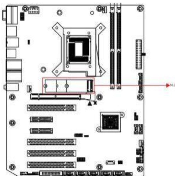
图 5-15 M.2 接口
