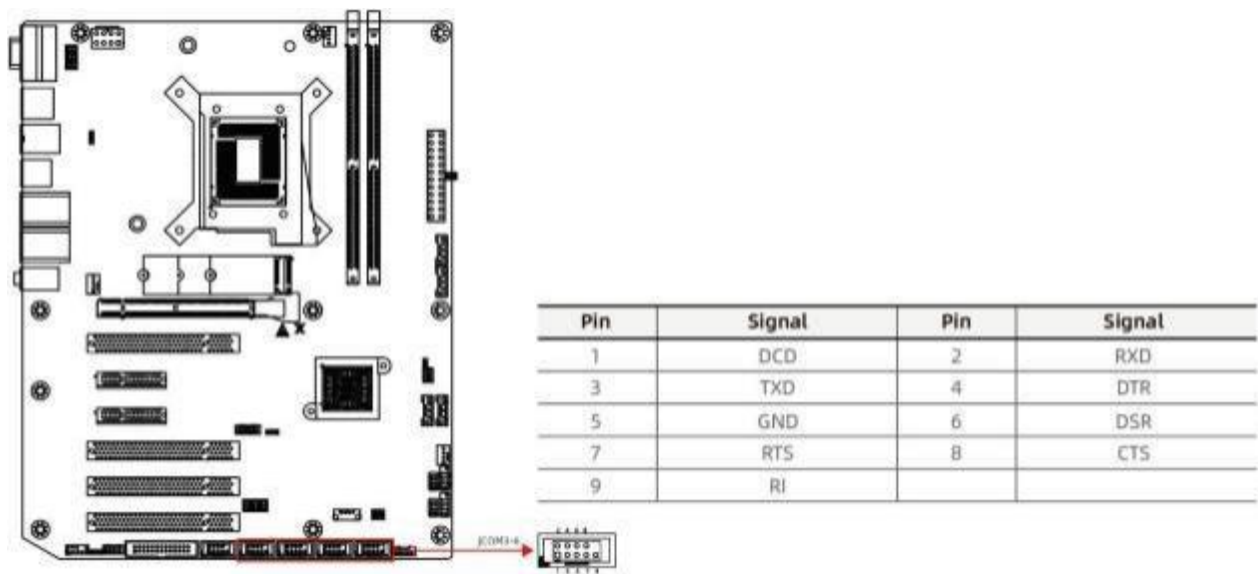
图 5-6 JCOM2-6 接口
