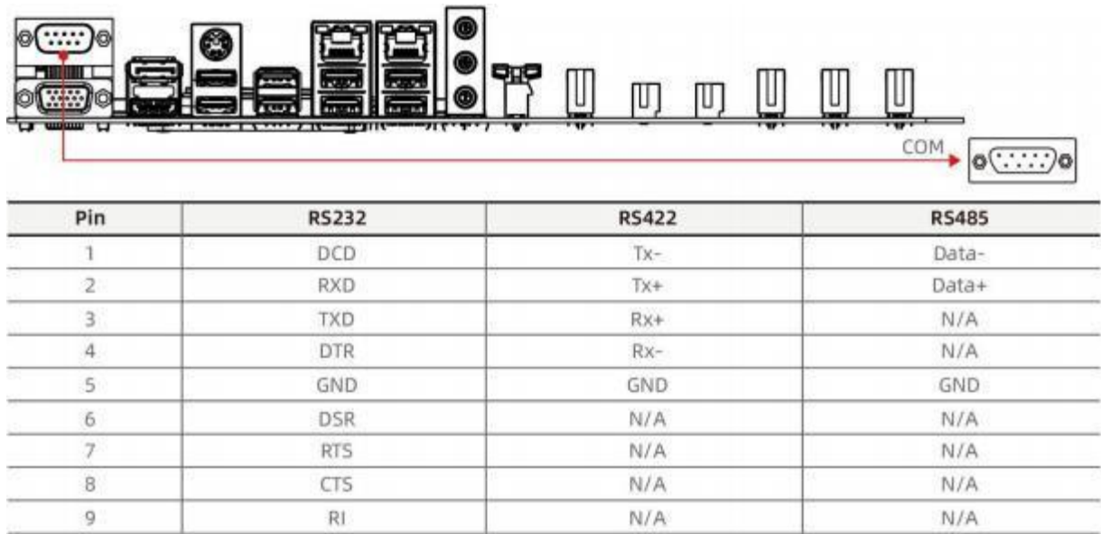
图 4-1 COM 接口
