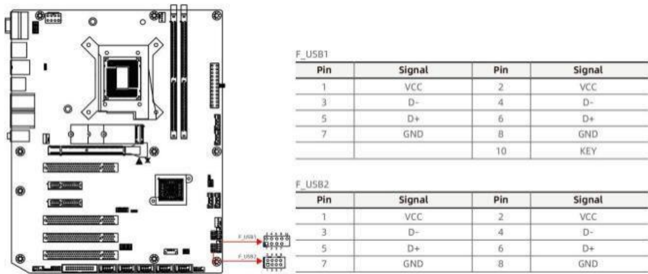
图 5-10 F_USB1/2 接口
