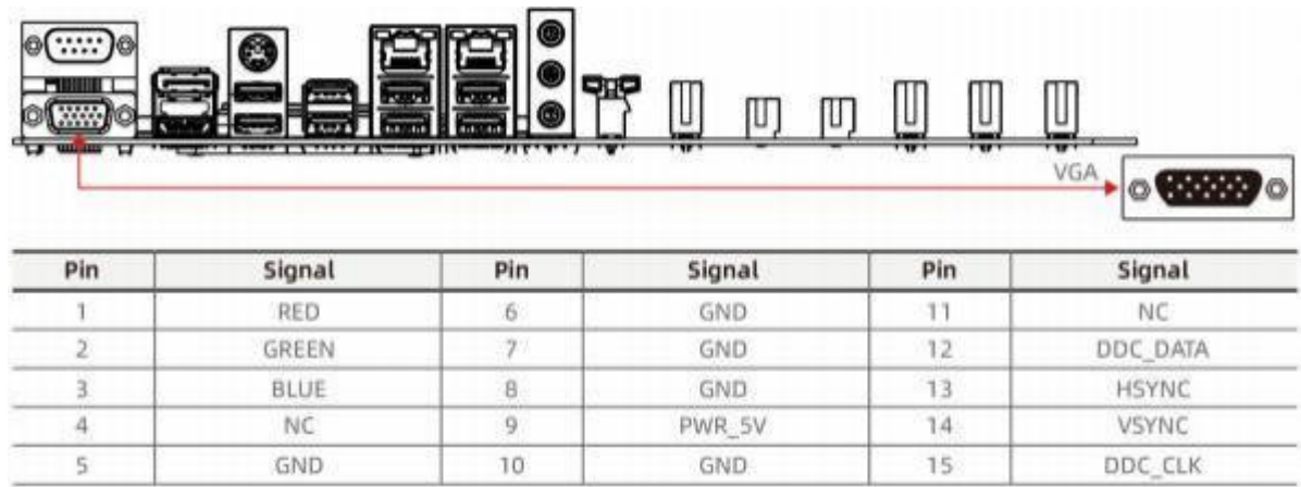
图 4-2 VGA 接口
