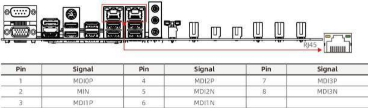
图 4-7 RJ45 接口
