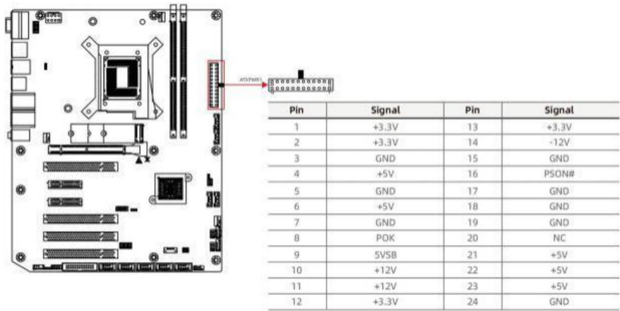
图 5-2 主板供电接口
