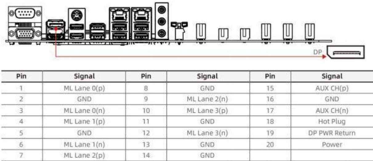
图 4-3 DP 接口
