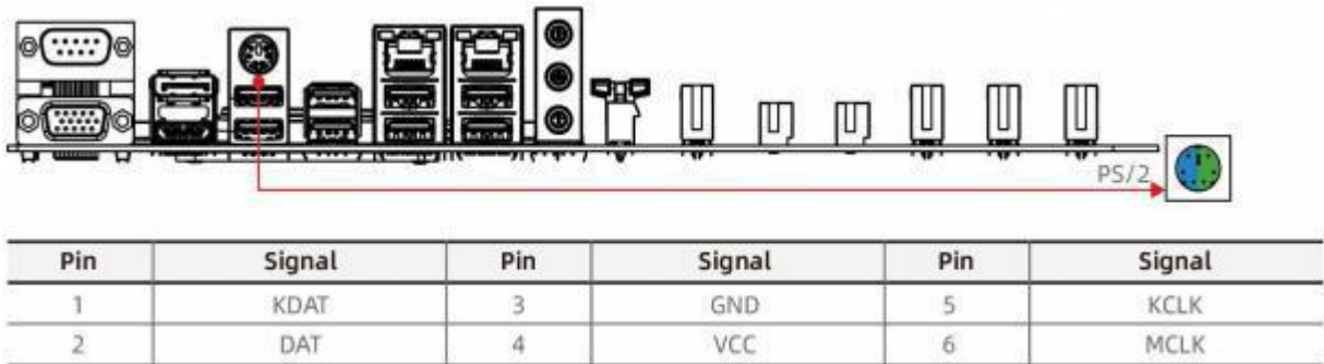
图 4-5 PS/2 接口
