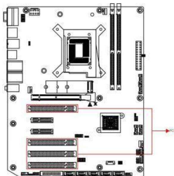
图 5-14 PCI 接口
