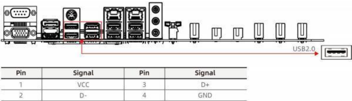
图 4-6 USB2.0 接口
