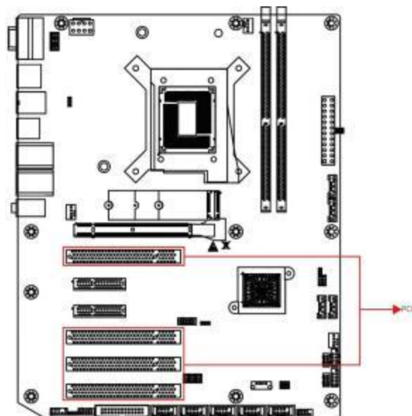
图 5-14 PCI 接口
