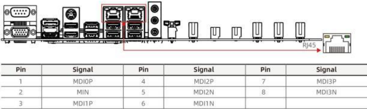
图 4-7 RJ45 接口
