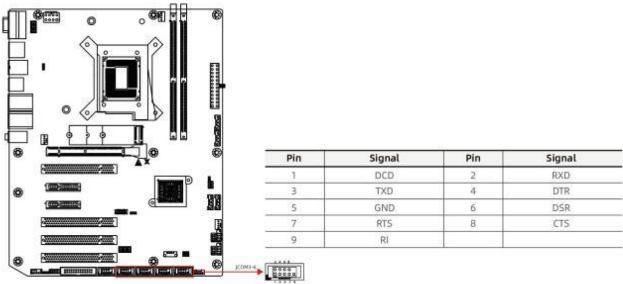
图 5-6 JCOM2-6 接口
