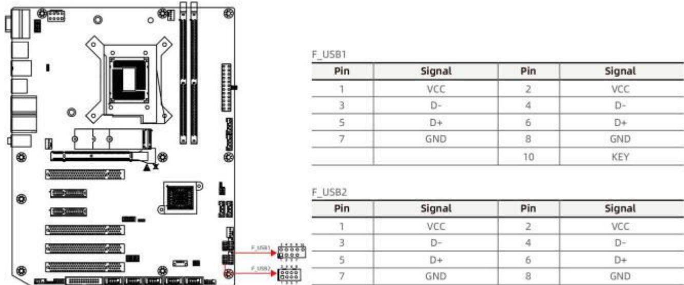
图 5-10 F_USB1/2 接口
