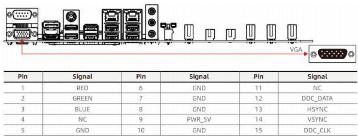
图 4-2 VGA 接口
