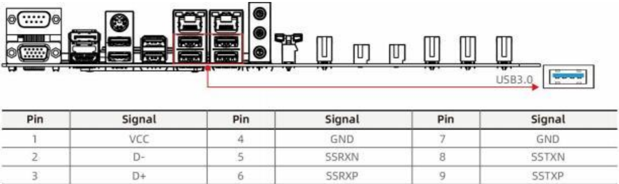
图 4-8 USB3.0 接口
