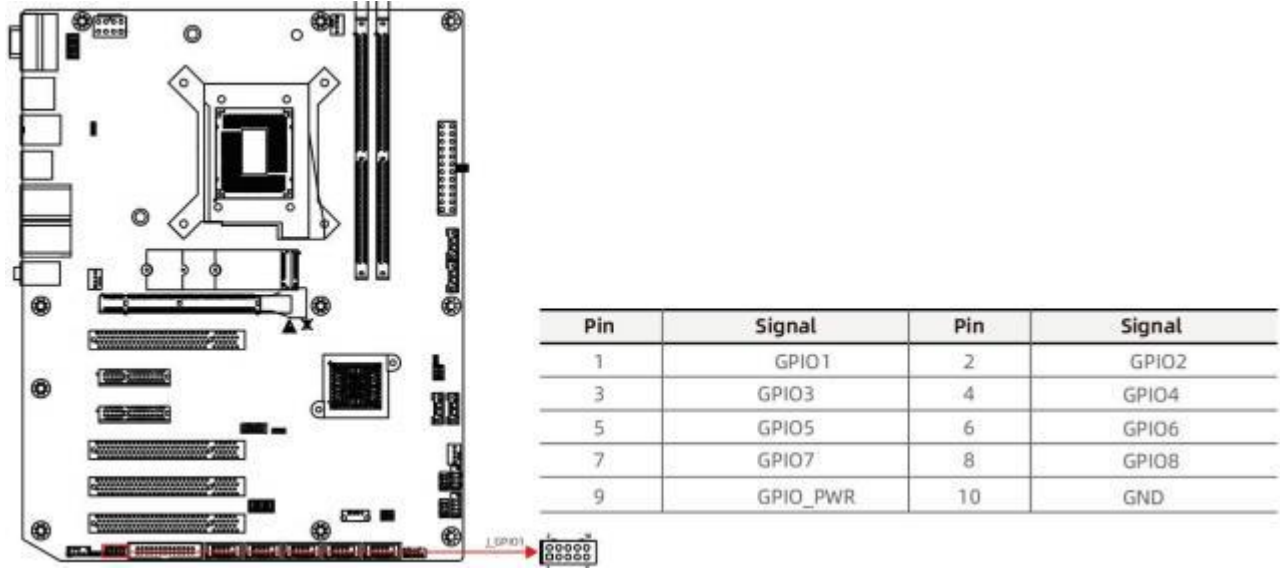
图 5-12 J_GPIO1 接口
