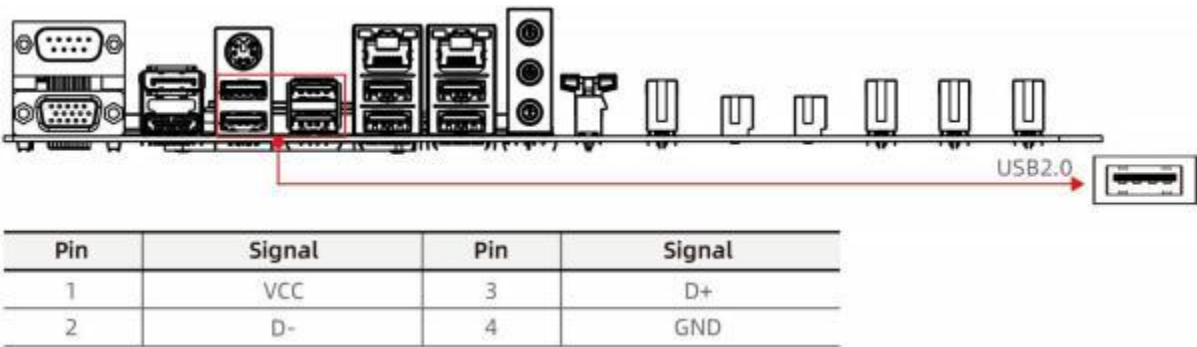
图 4-6 USB2.0 接口
