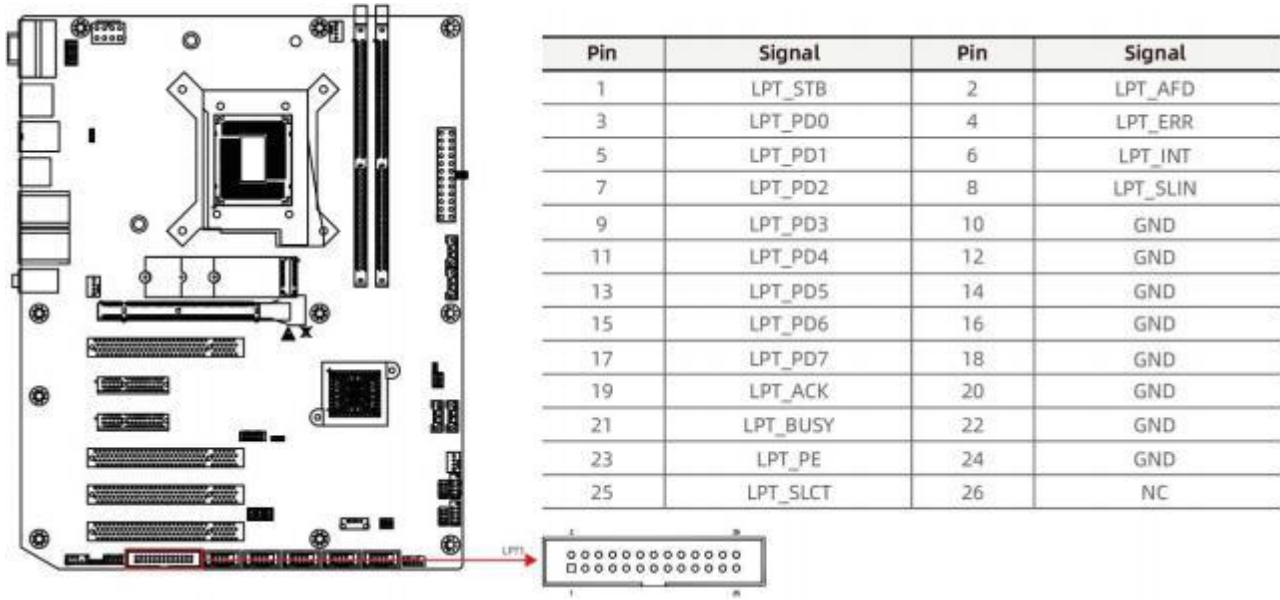
图 5-11 LPT1 接口
