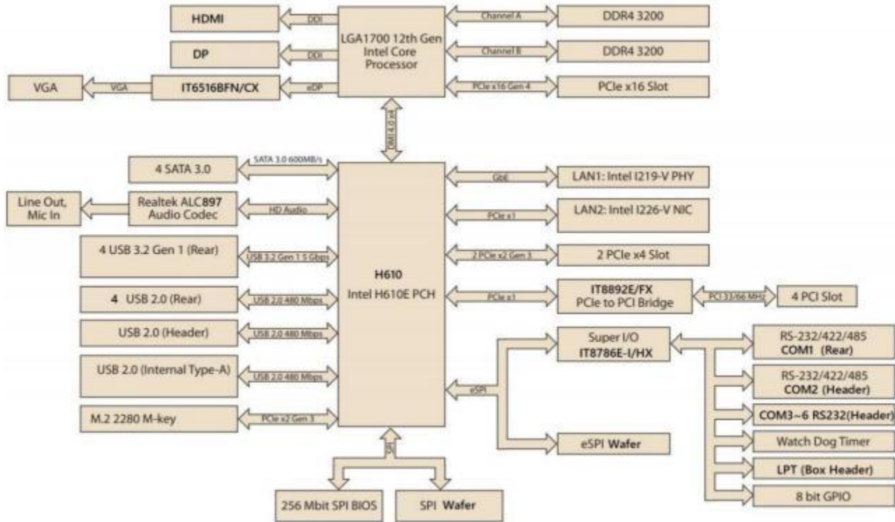
图 2-1 主板架构图
