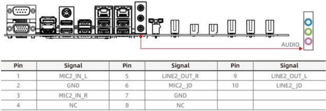
图 4-9 音频接口
