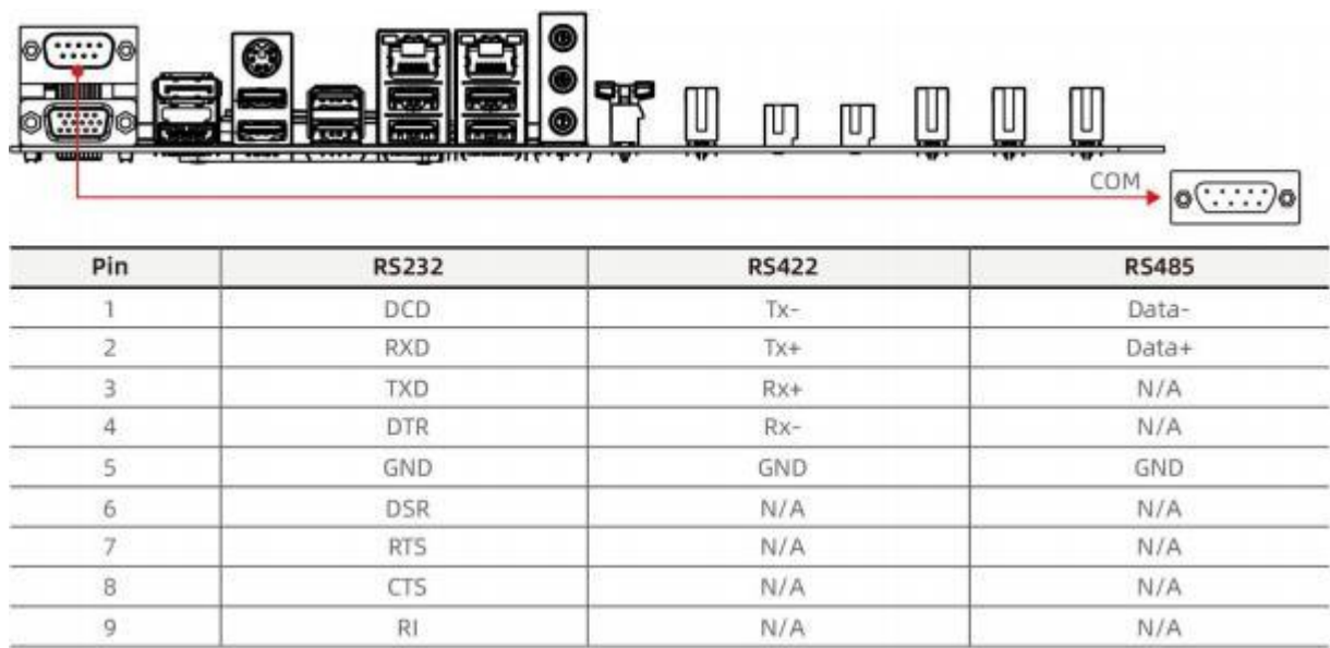
图 4-1 COM 接口
