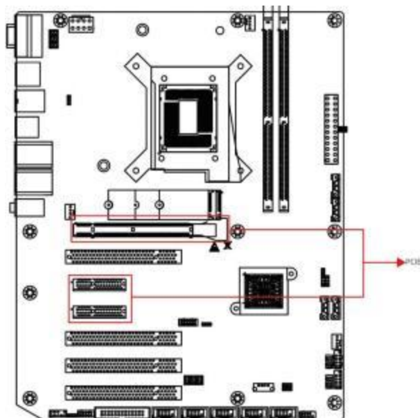
图 5-13 PCIe 接口
