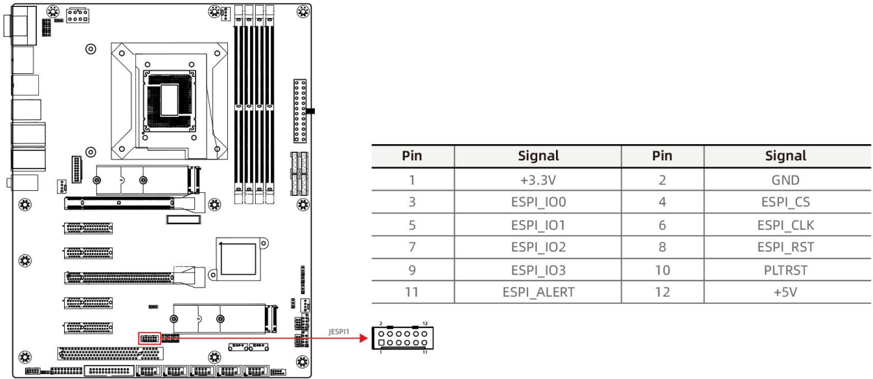
图 5-11 JESPI1 接口
