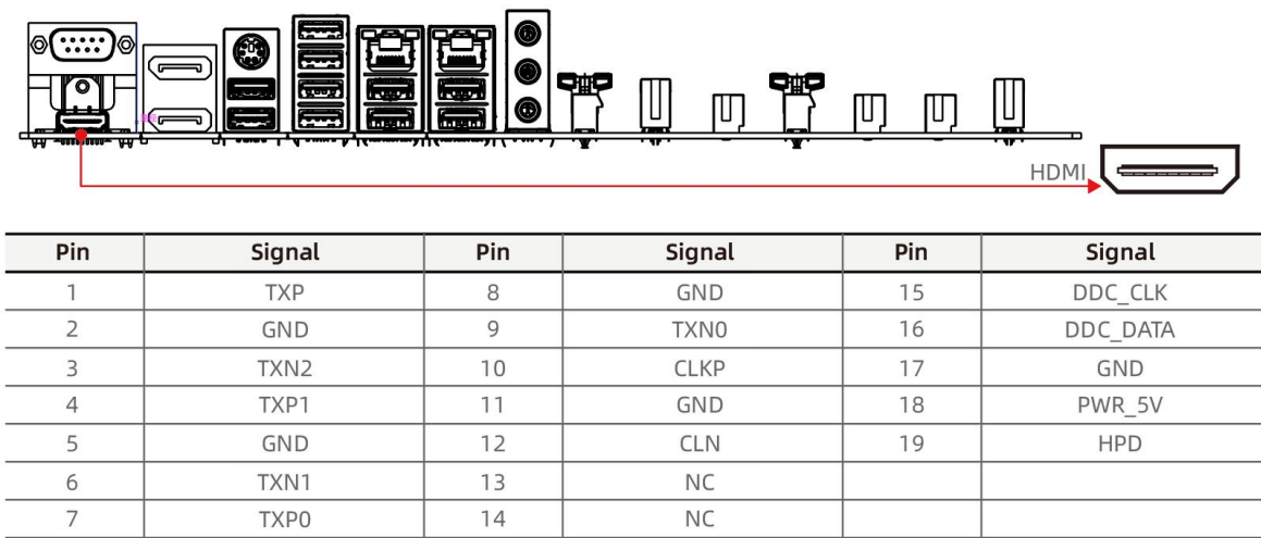
图 4-2 HDMI 接口
