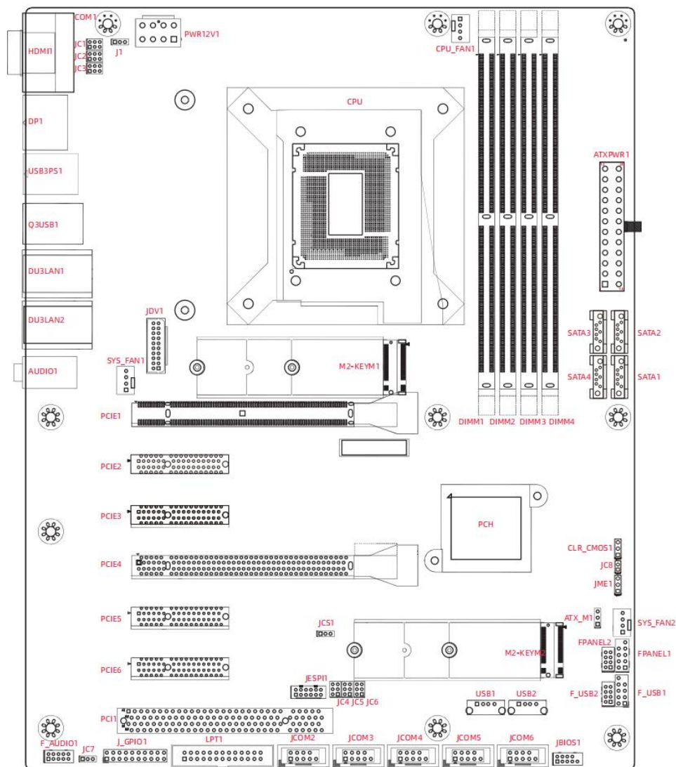
图 2-3 主板布局图
