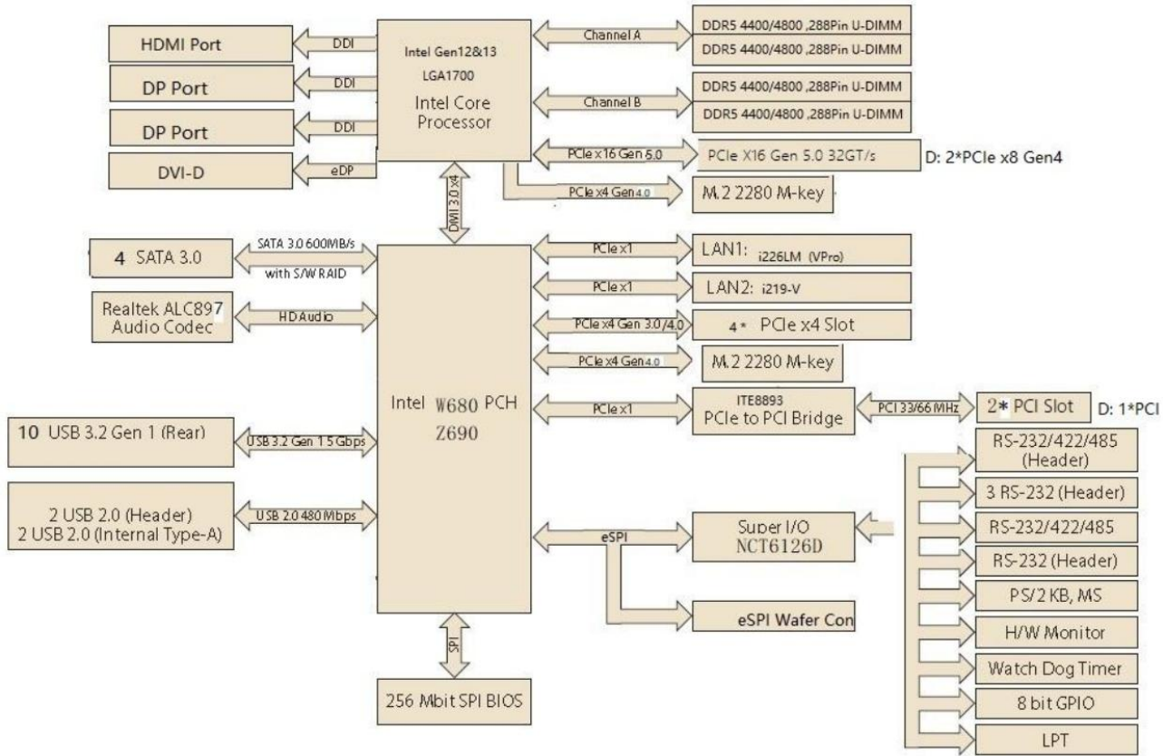
图 2-1 主板架构图
