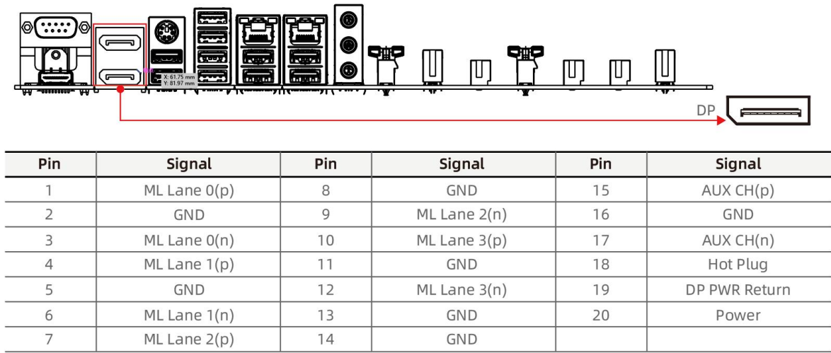
图 4-3 DP 接口
