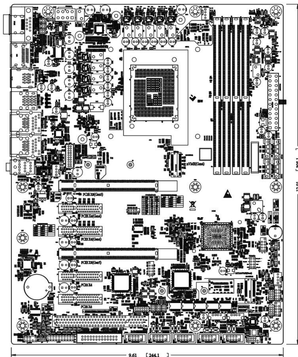
图 2-4 主板尺寸图
