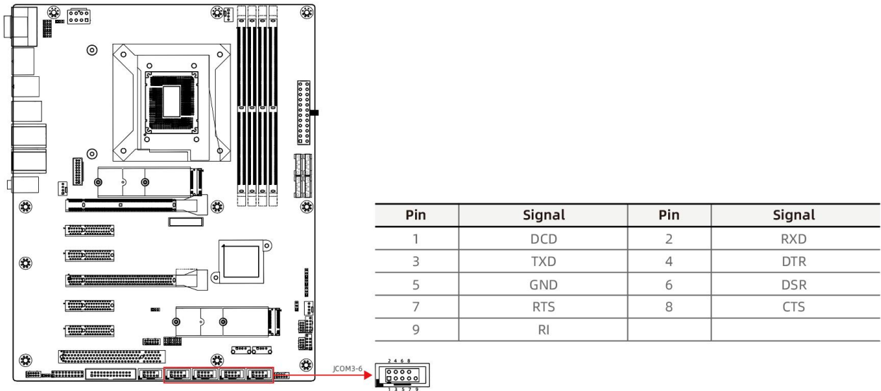
图 5-6 JCOM3-6 接口
