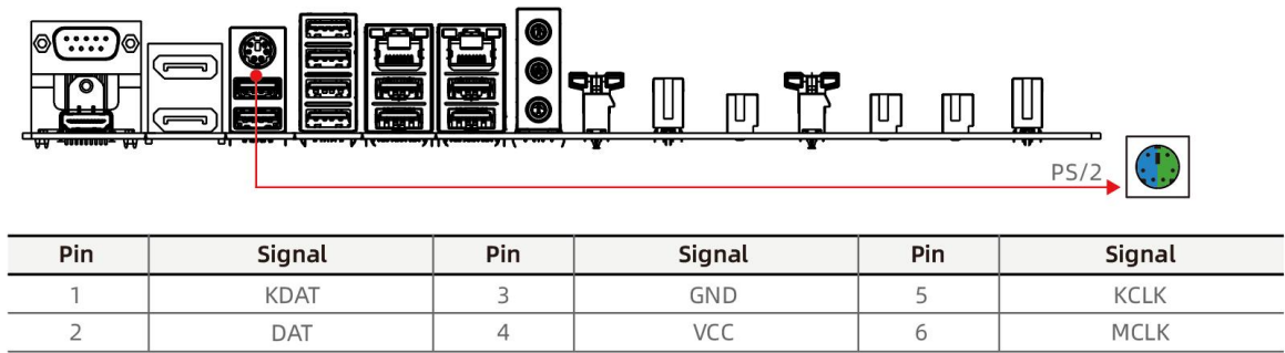
图 4-4 PS/2 接口
