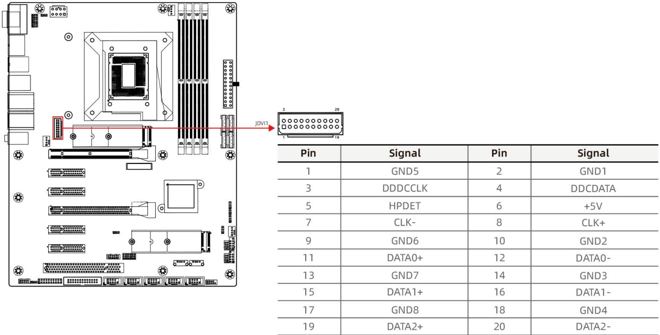
图 5-13 DVI1 接口
