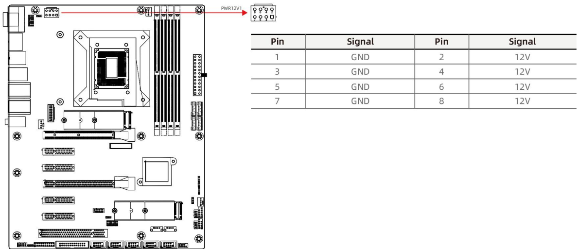
图 5-1 CPU 供电接口
