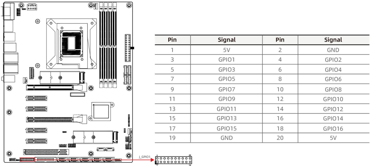
图 5-14 J_GPIO1 接口
