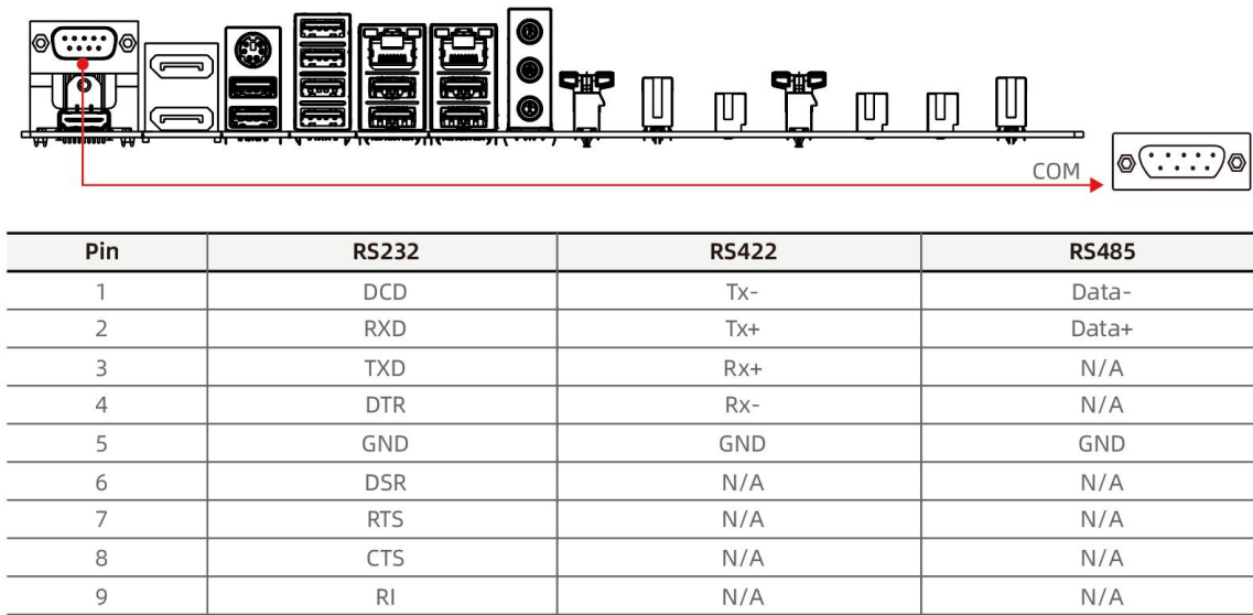
图 4-1 COM 接口
