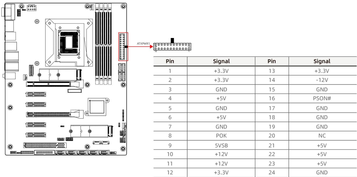
图 5-2 主板供电接口
