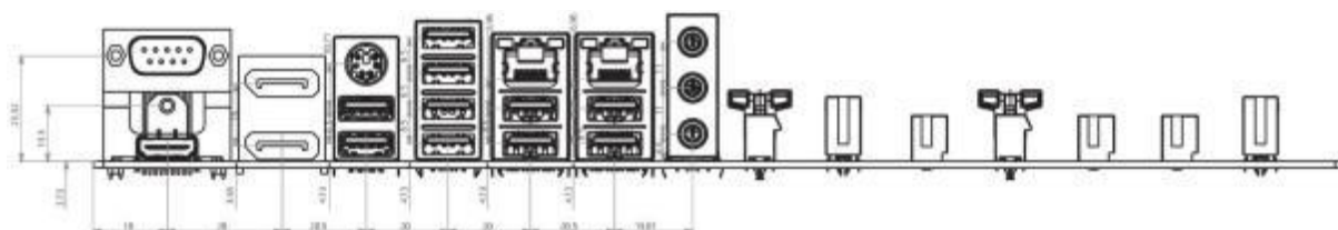
图 2-2 主板 IO 接口结构图
