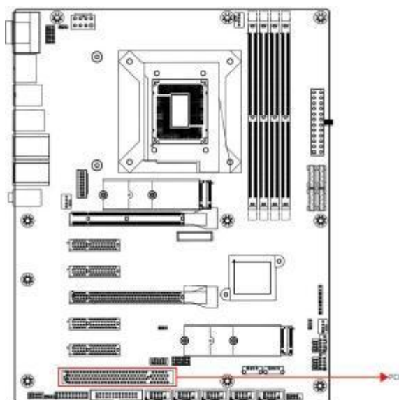
图 5-16 PCI 接口
