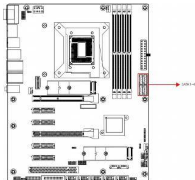
图 5-18 SATA 接口
