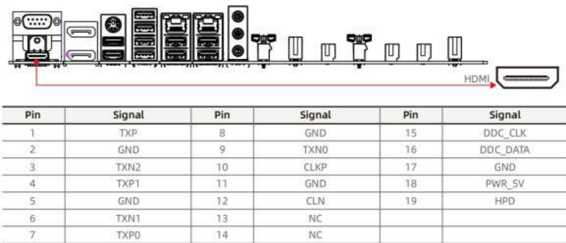
图 4-2 HDMI 接口
