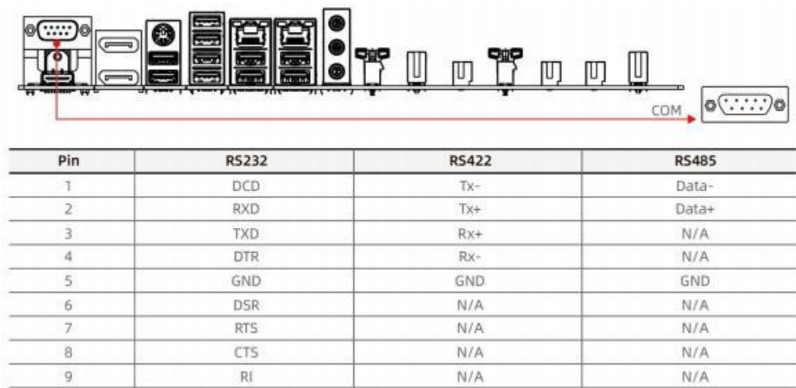
图 4-1 COM 接口
