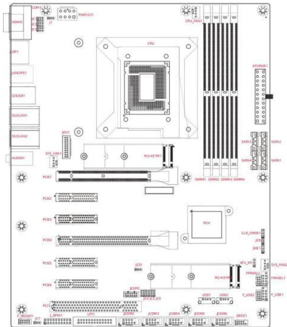
图 2-3-1 主板布局图
