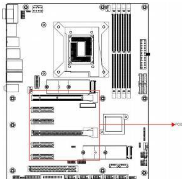
图 5-15 PCIe 接口
