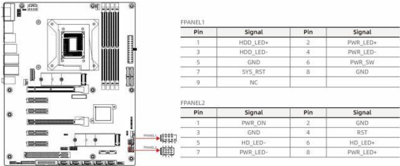
图 5-9 前置面板控制信号 FPANEL1-2 接口
