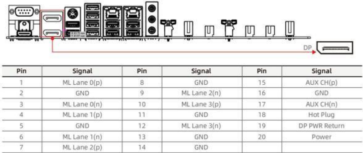
图 4-3 DP 接口
