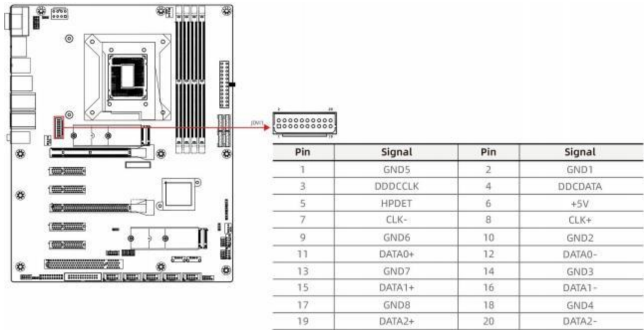
图 5-13 DVI1 接口
