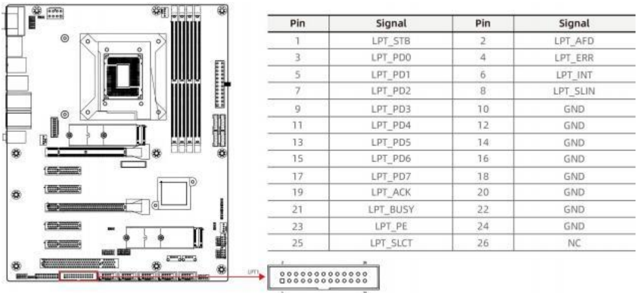
图 5-12 LPT1 接口
