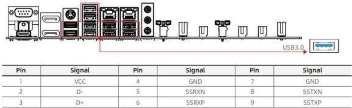
图 4-5 USB3.0 接口
