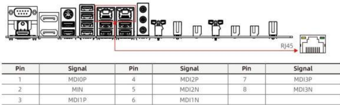
图 4-6 RJ45 接口
