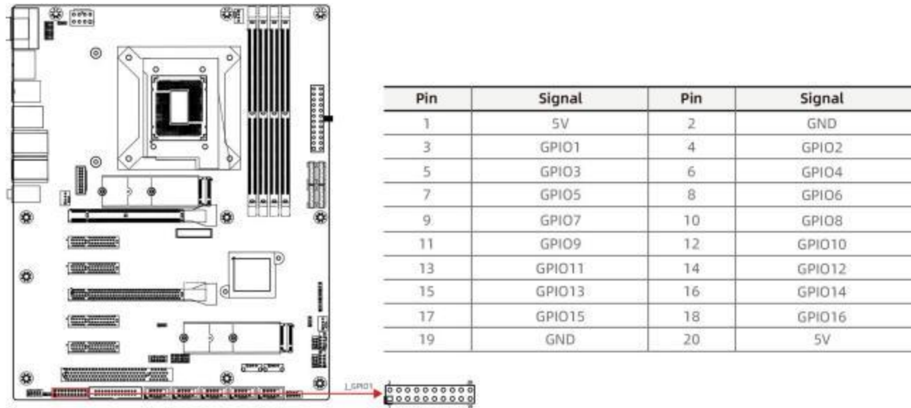
图 5-14 J_GPIO1 接口
