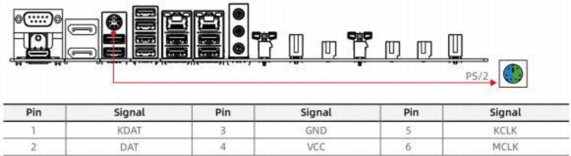
图 4-4 PS/2 接口
