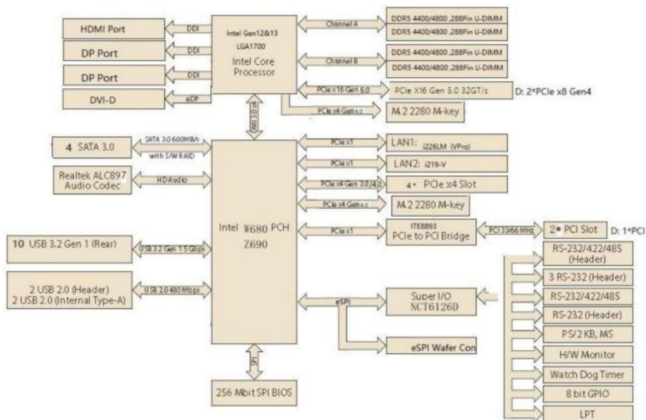
图 2-1 主板架构图
