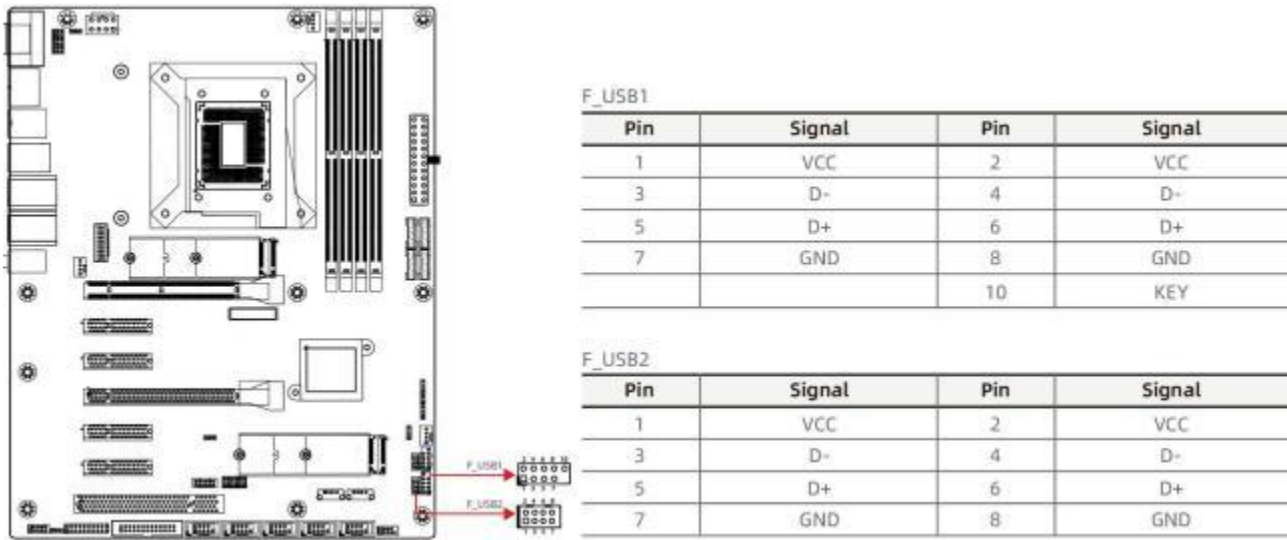
图 5-10 F_USB1-2 接口
