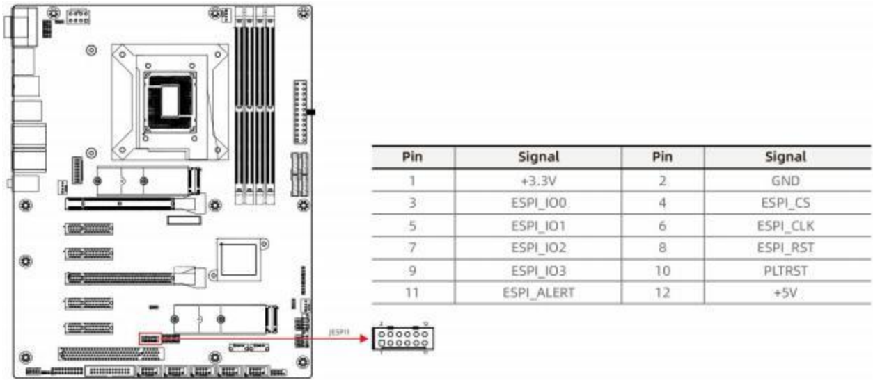
图 5-11 JESPI1 接口
