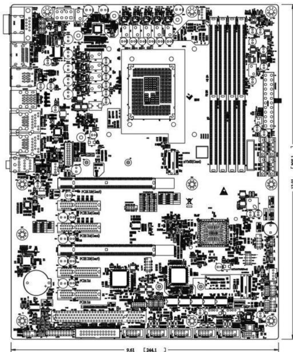
图 2-4 主板尺寸图
