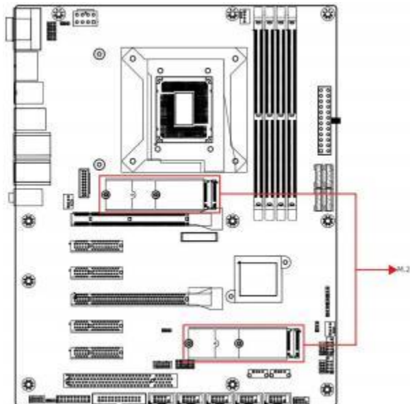
图 5-17 M.2接口
