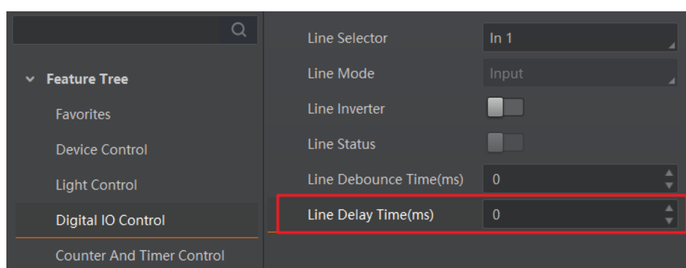
图5-20 触发延迟设置
