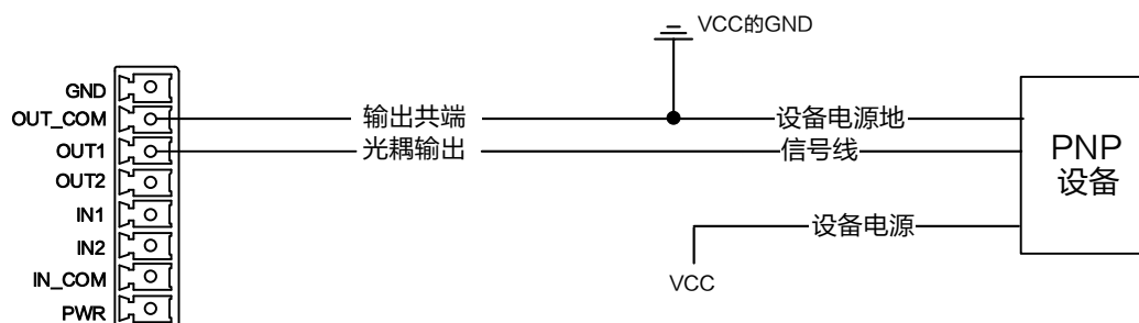
图4-11 输出信号接 PNP 设备（方式1）
