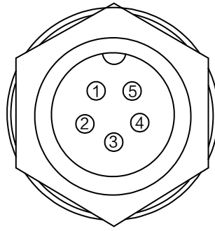
图4-16 12M-5F 接口外观
