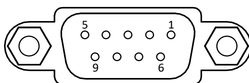
图4-4 9-pin 母头连接器
