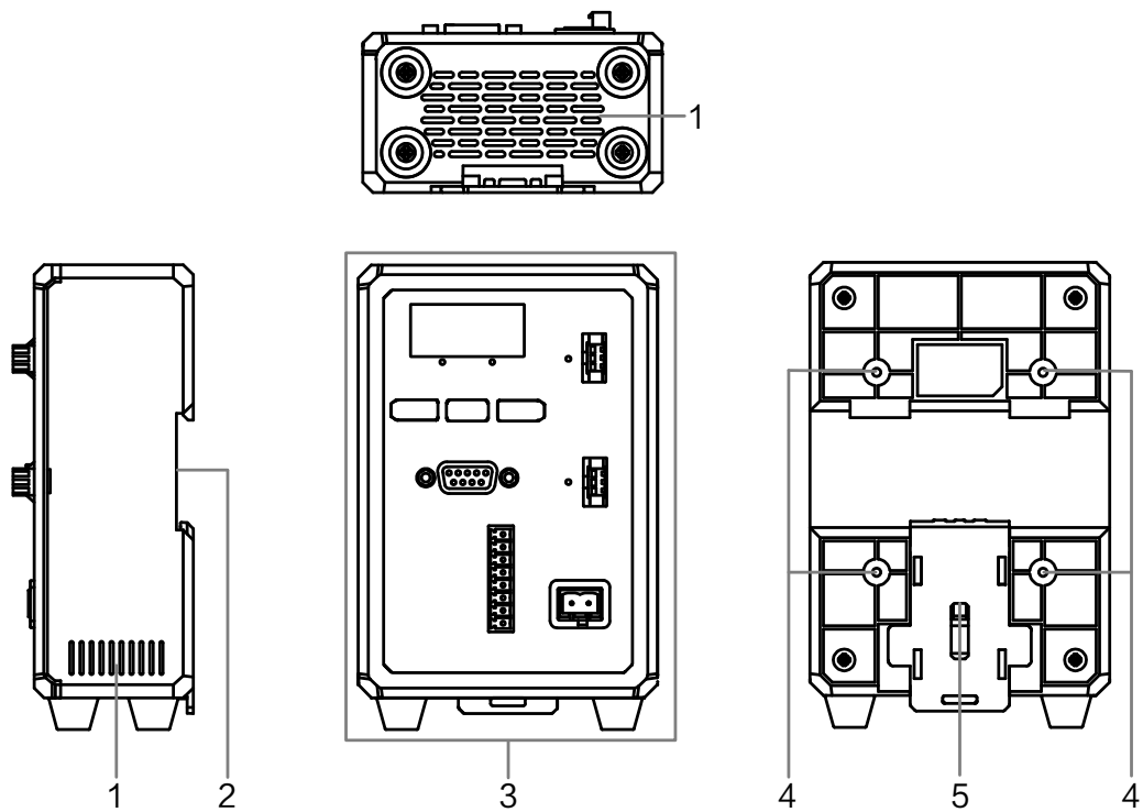
图2-1 设备产品外观
