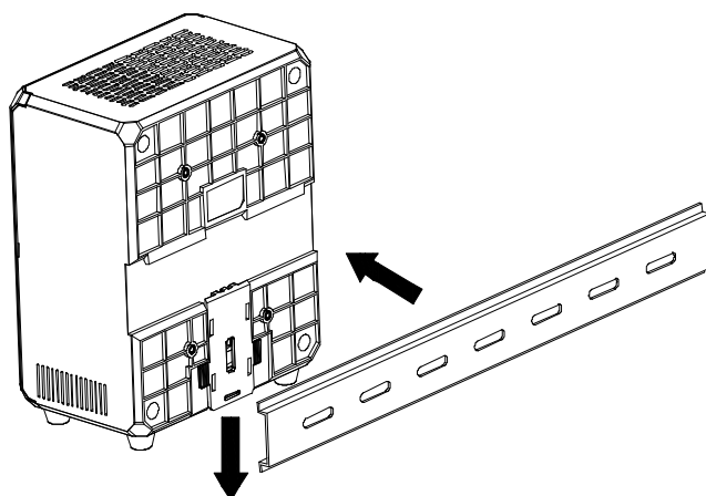
图3-1 导轨卡入设备
