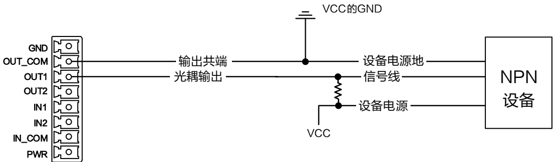
图4-14 输出信号接 NPN 设备（使用外接上拉电阻）
