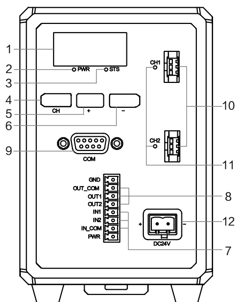
图4-1 10 W 设备面板界面介绍
