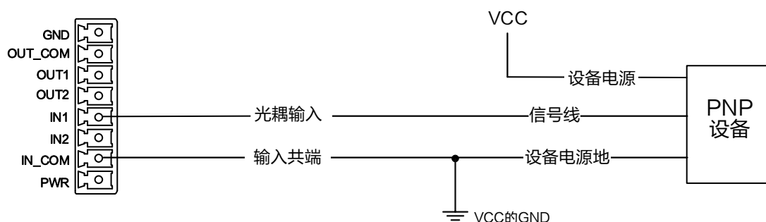
图4-6 输入信号接 PNP 设备（方式1）
