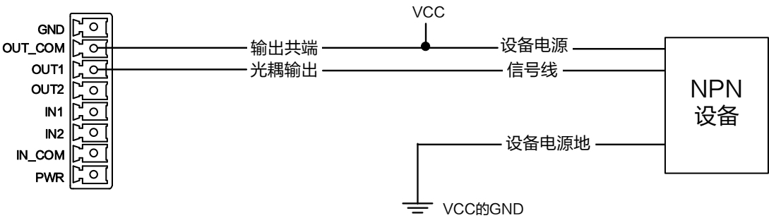
图4-13 输出信号接 NPN 设备（不使用上拉电阻）
