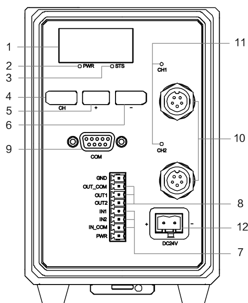
图4-2 30 W 设备面板界面介绍
