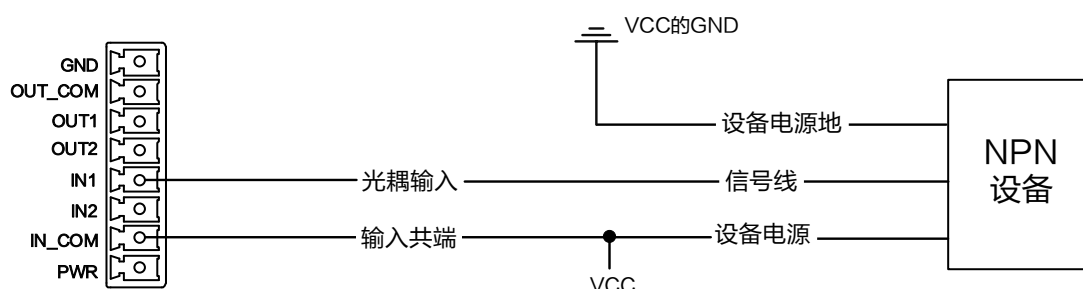
图4-8 输入信号接 NPN 设备（不使用外接电阻）
