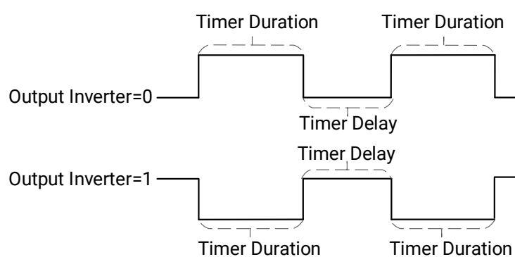
图5-12 定时器输出原理
