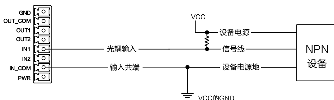
图4-9 输入信号接 NPN 设备（使用外接上拉电阻）
