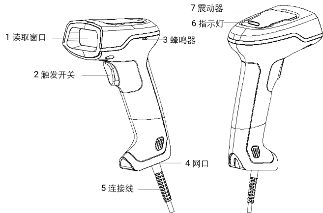
图2-1 紧凑型设备外观
