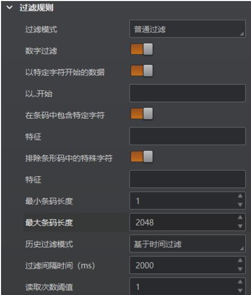
图6-10 过滤规则参数
