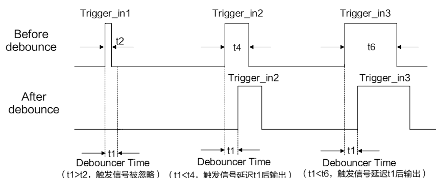
图6-33 触发输入信号去抖时序
