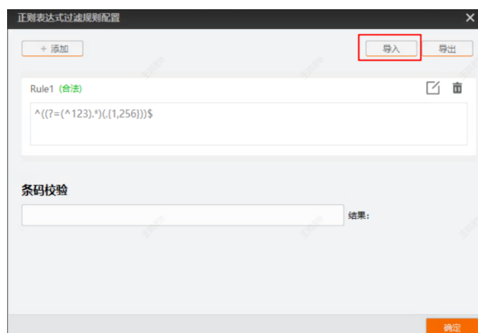
图6-11 正则表达式过滤规则导入
