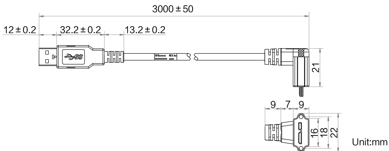
MV-ACU3-MBMs(down)-AM-ST-3m:
