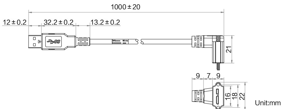
MV-ACU3-MBMs(down)-AM-ST-1m:
