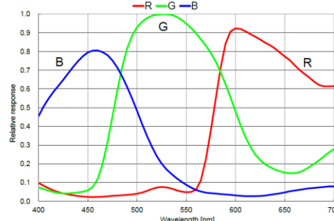
MV-CS060-10GC 量子效率
