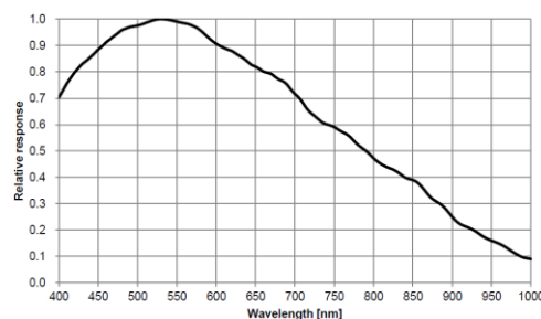
MV-CS060-10GM 量子效率
