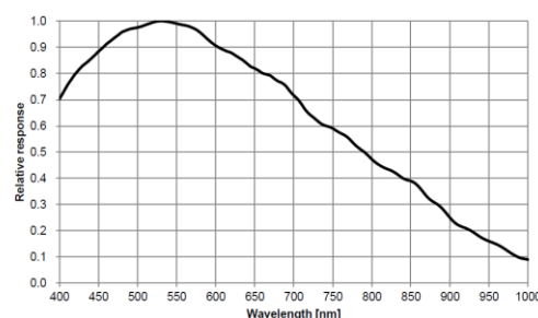
MV-CS060-10GM V5 量子效率
