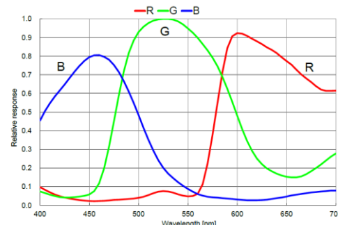
MV-CS060-10GC V5 量子效率
