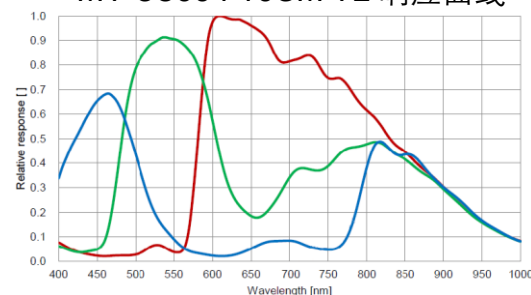
MV-CU004-10GC V2 响应曲线
