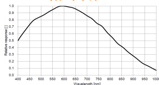
MV-CU004-10GM V2 响应曲线
