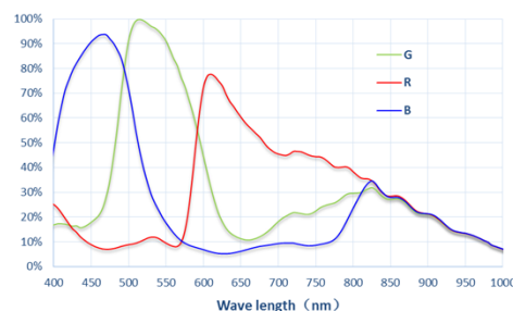
MV-CU013-80GC V2 响应曲线
