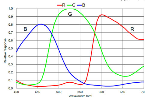
MV-CU060-10GC V2 响应曲线
