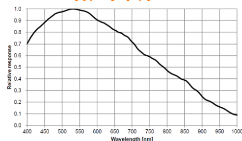
MV-CU060-10GM V2 响应曲线
