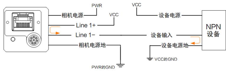
图 7-12 Line 1 接 NPN 设备（不使用上拉电阻）
