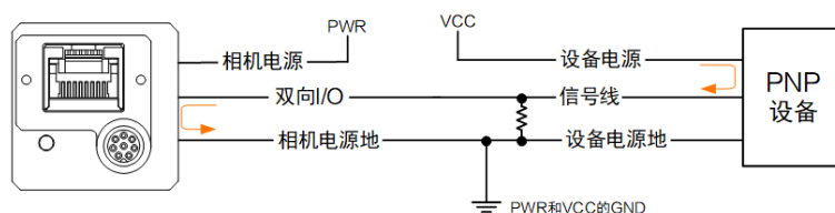
图 7-14 Line 2 作为输入接 PNP 设备
