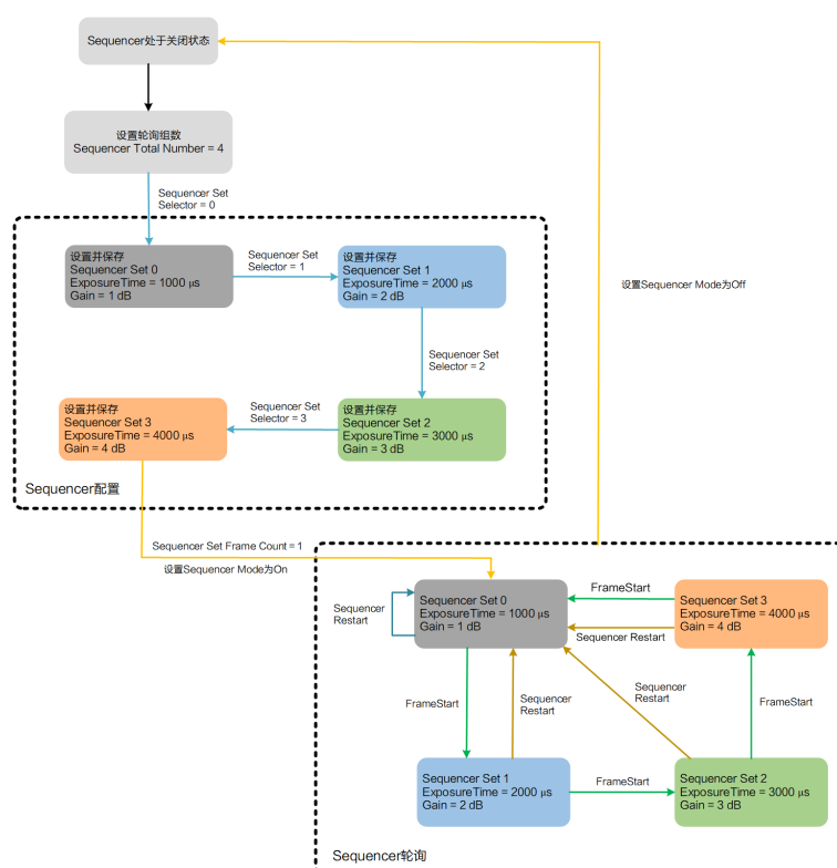
图 12-1 Sequencer 轮询
