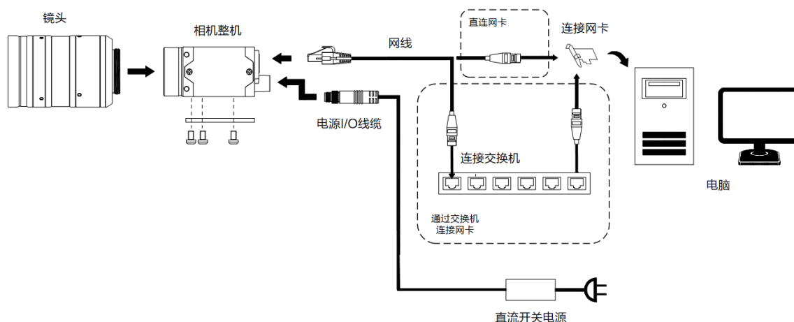
图 6-2 连接 BASE 版本相机
