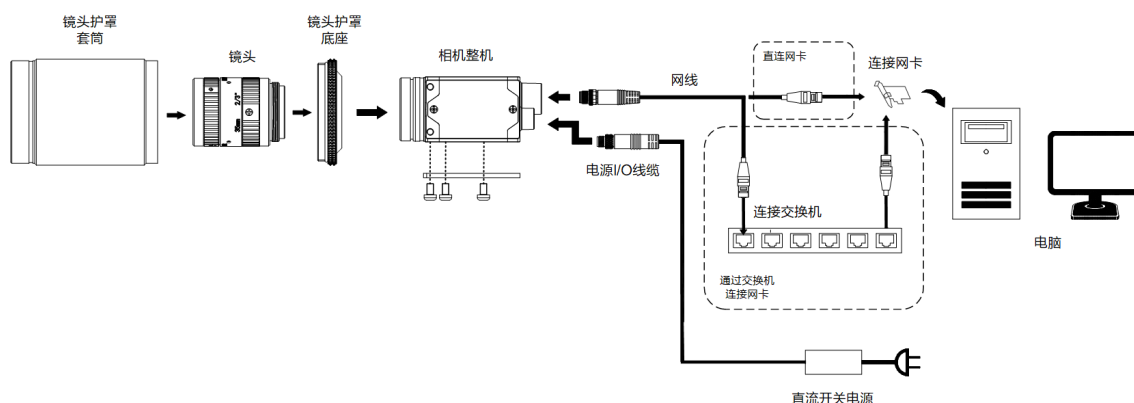
图 6-3 连接 PRO 版本相机
