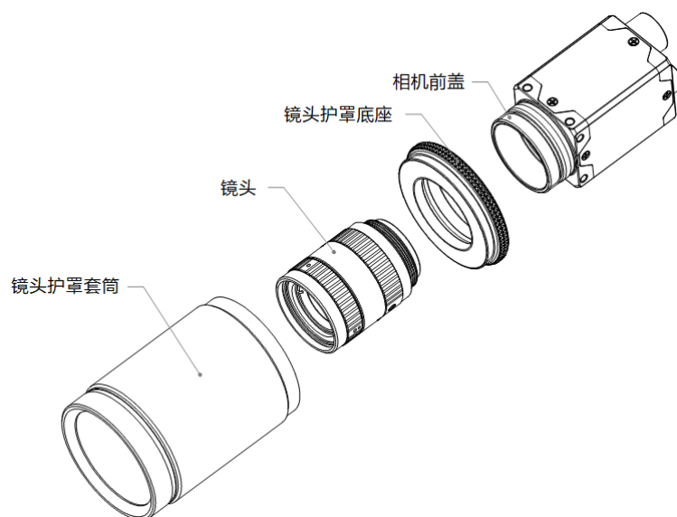
图 6-4 安装镜头与镜头护罩
