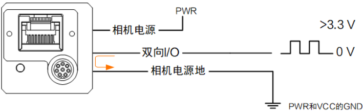
图 7-16 Line 2 作为输入接开关
