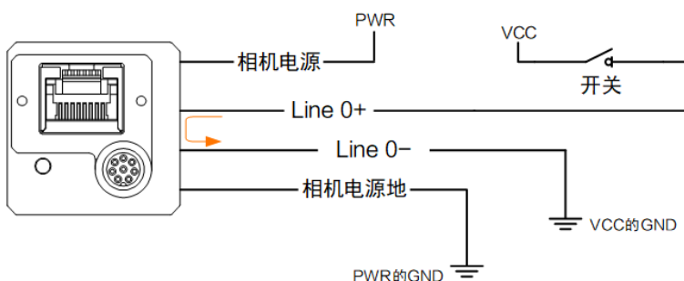
图 7-10 Line 0 接开关
