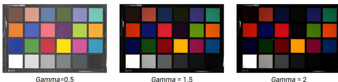
图 12-5 Gamma 效果示例
