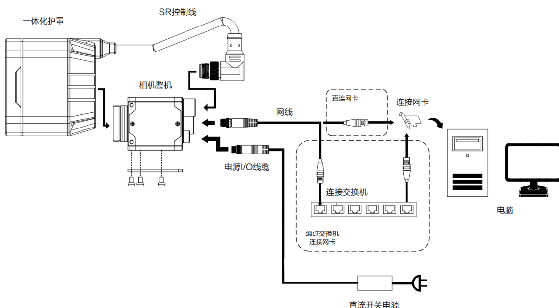
图 6-5 连接 MAX 版本相机
