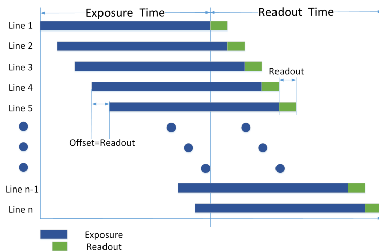
图 9-2 卷帘快门
