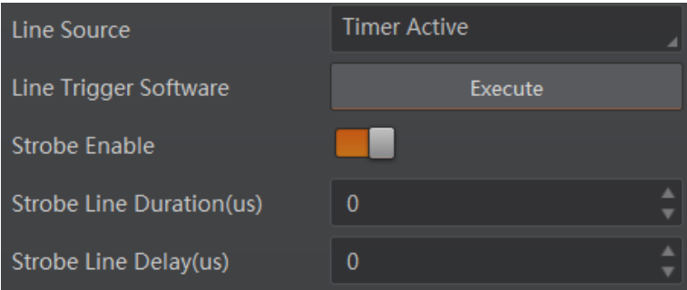
图 8-11 Timer Active 相关参数
