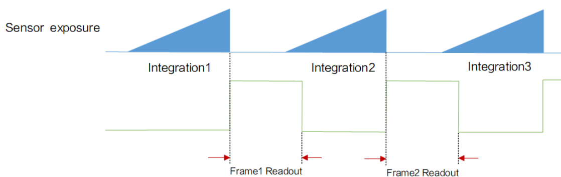
图 9-9 内触发模式
