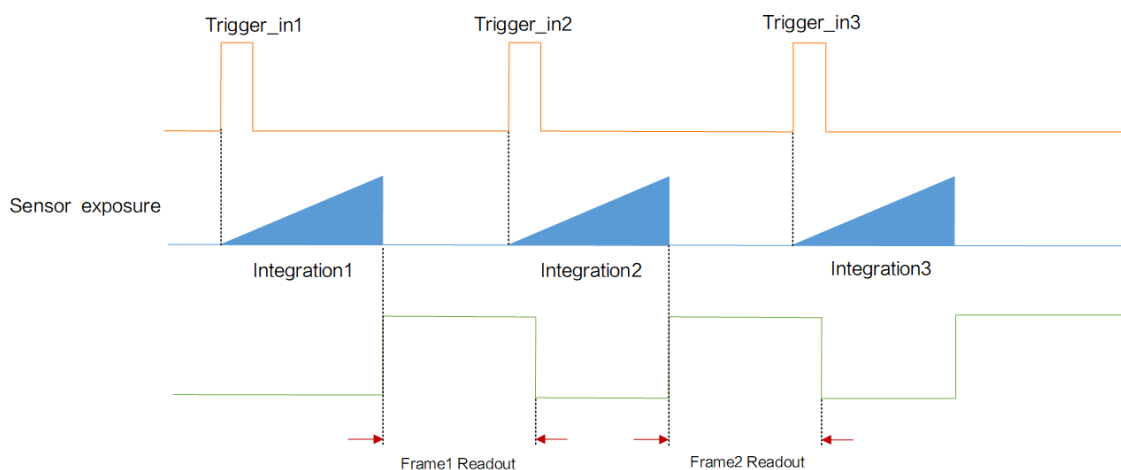
图 9-10 外触发模式
