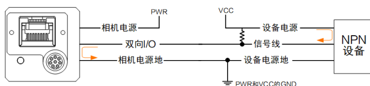
图 7-15 Line 2 作为输入接 NPN 设备
