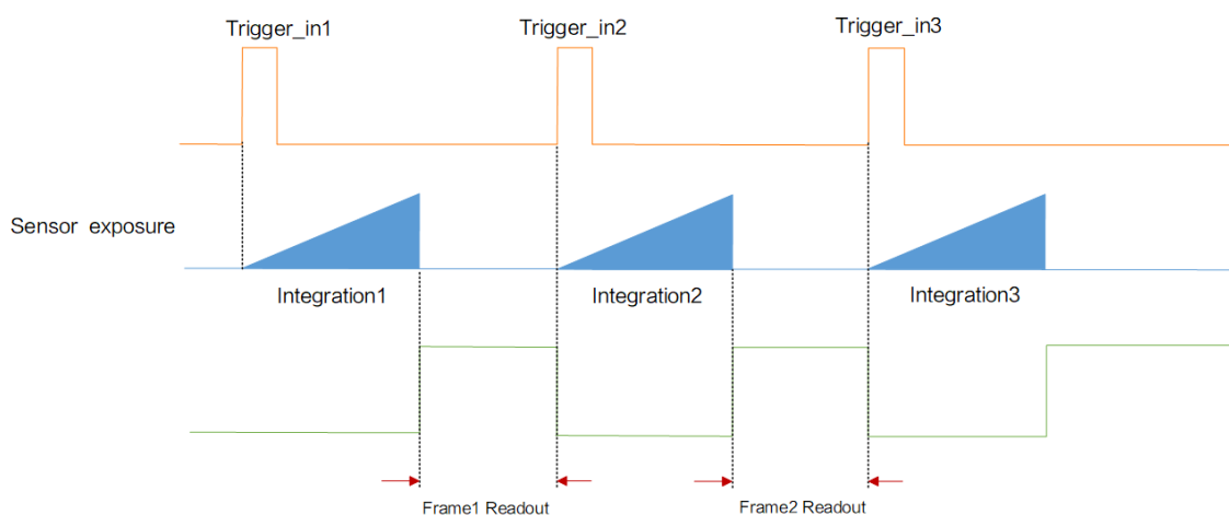
图 9-8 外触发模式
