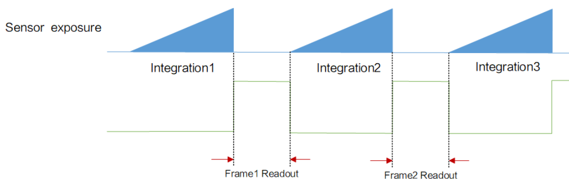
图 9-7 内触发模式
