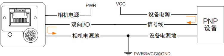
图 7-17 Line 2 作为输出接 PNP 设备
