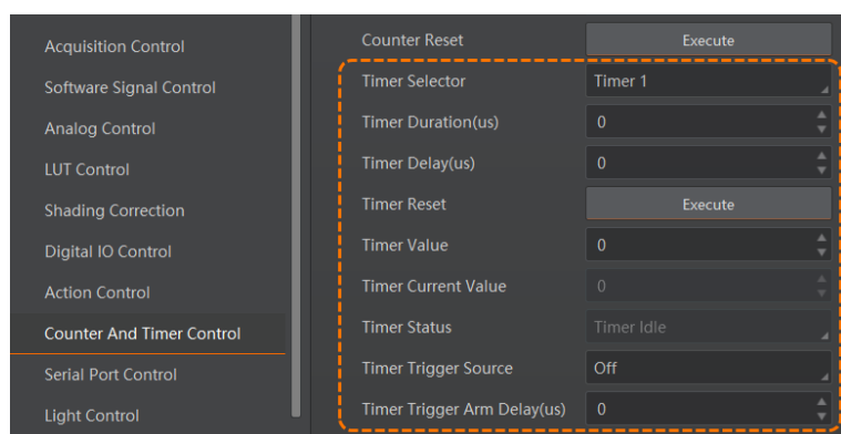
图 8-13 定时器相关参数
