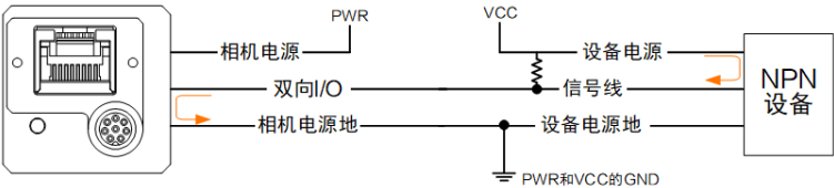
图 7-18 Line 2 作为输出接 NPN 设备
