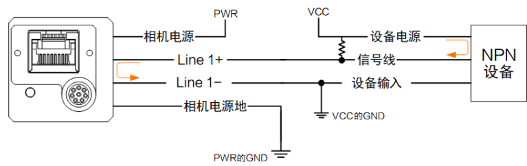
图 7-13 Line 1 接 NPN 设备（使用上拉电阻）
