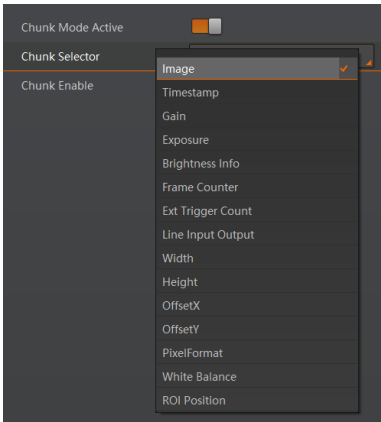
图 13-4 选择嵌入的信息
