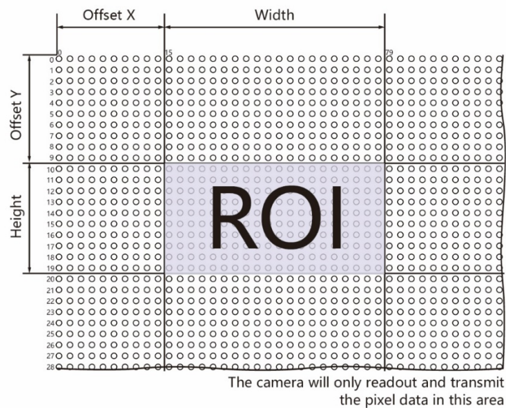
图 11-2 ROI 区域
