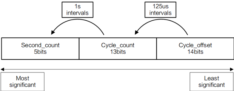
图 13-2 Timestamp 数据格式
