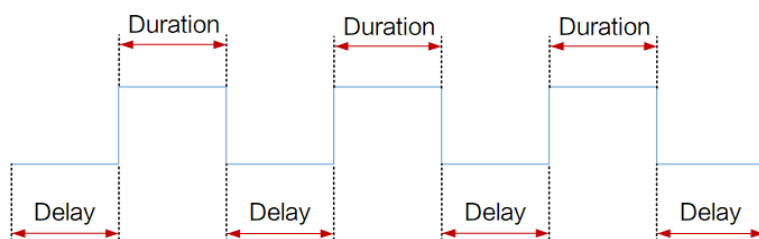
图 8-12 Timer Active 时序图
