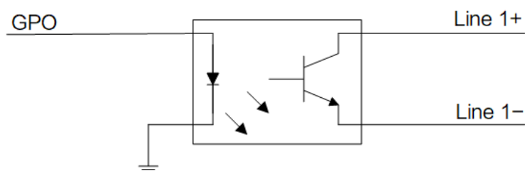
图 7-3 光耦隔离输出内部电路
