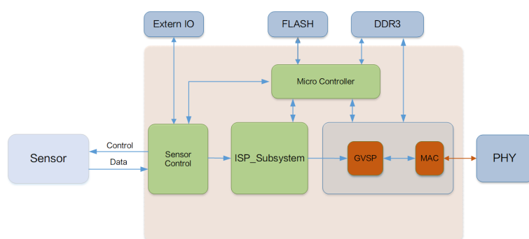
图 3-1 工作原理
