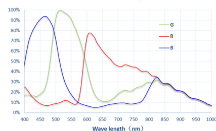
MV-CE013-80GC 响应曲线
