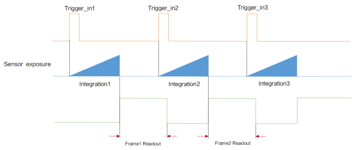
图 9-7 外触发模式
