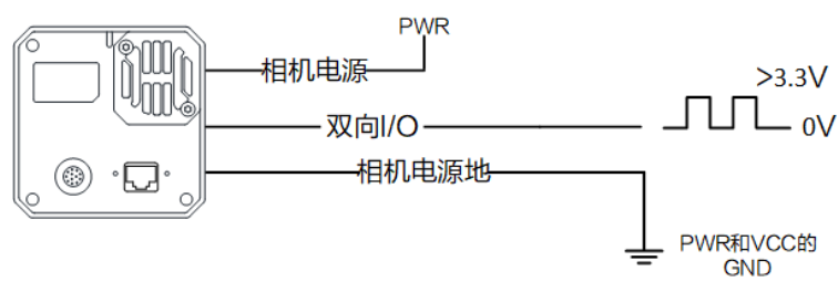
图 7-15 Line 2 作为输入接开关
