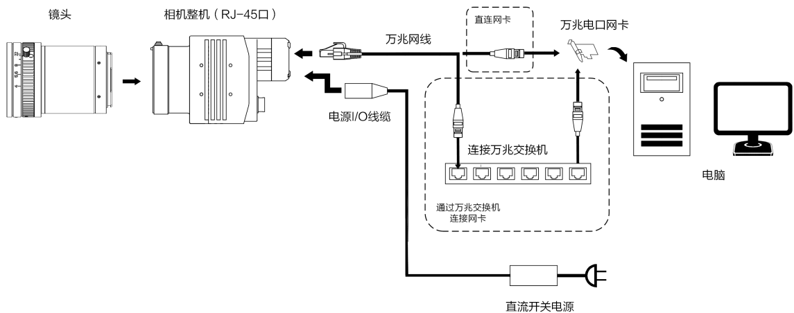
图 6-2 连接万兆 RJ-45 口相机
