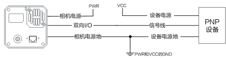
图 7-16 Line 2 作为输出接 PNP 设备
