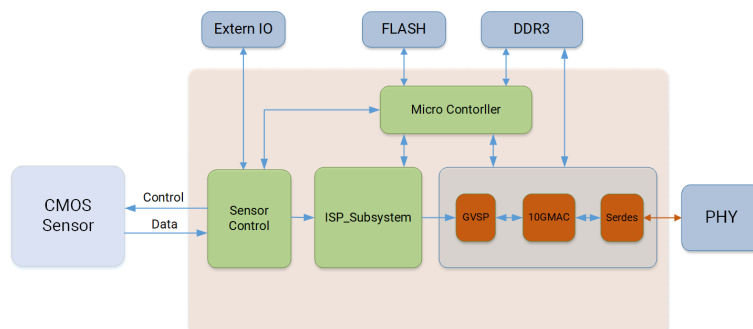
图 3-1 工作原理
