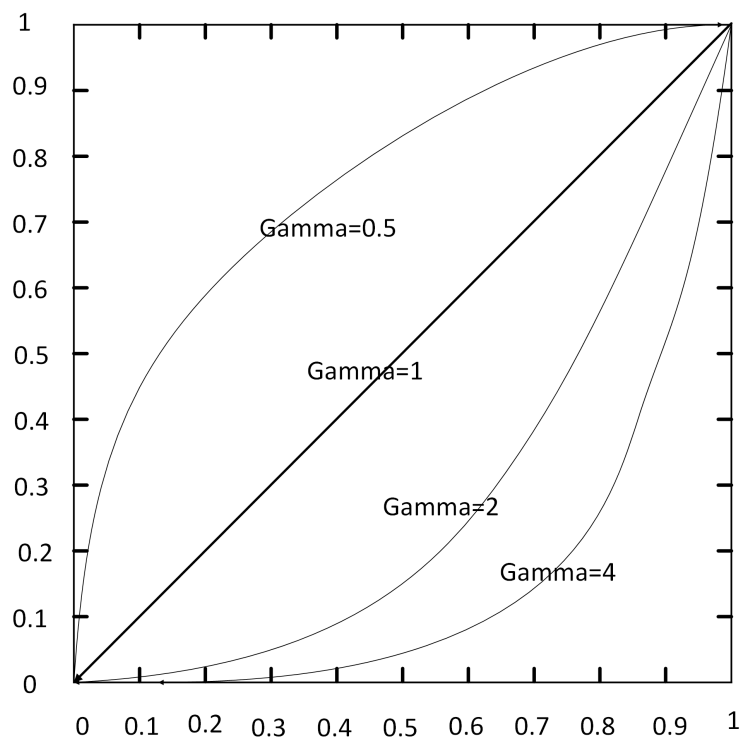
图 12-2 Gamma 曲线图
