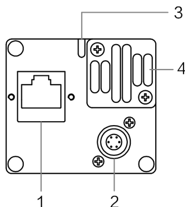
图 4-3 RJ-45 口、6-pin P7 接口、带风扇相机外观
