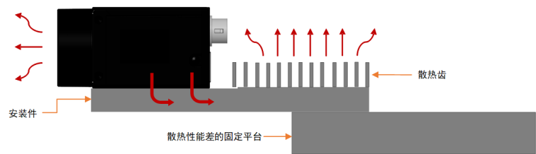
图 4-11 增加散热齿的安装件
