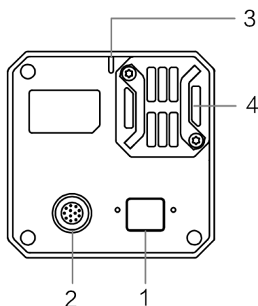
图 4-1 RJ-45 口、12-pin P10 接口、带风扇相机外观
