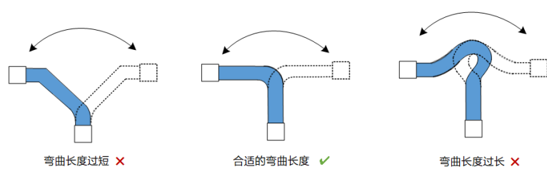
图 5-5 预留合适的弯曲长度
