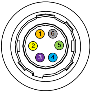
图 4-6 6-pin P7 接口
