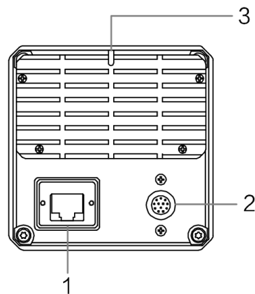
图 4-2 RJ-45 口、12-pin P10 接口、不带风扇相机外观
