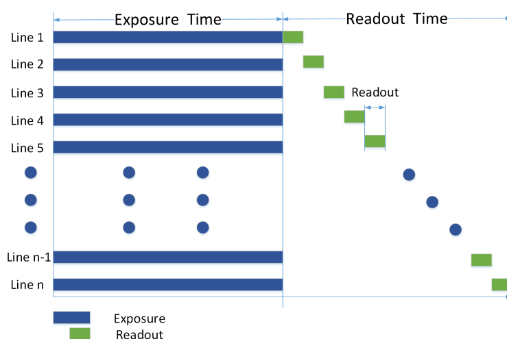
图 9-1 全局快门
