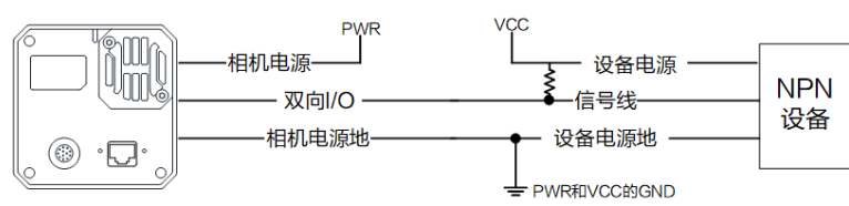
图 7-17 Line 2 作为输出接 NPN 设备
