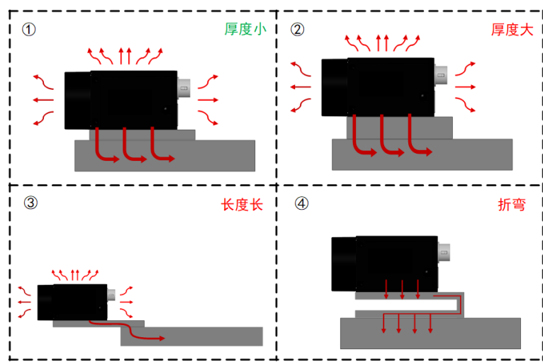
图 4-10 不同安装方式的导热路径
