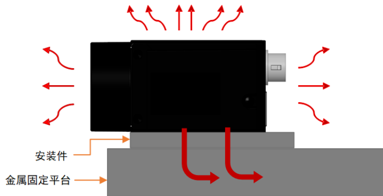
图 4-9 安装件散热
