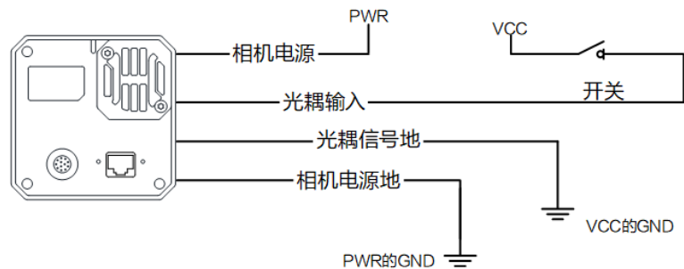
图 7-10 Line 0 接开关
