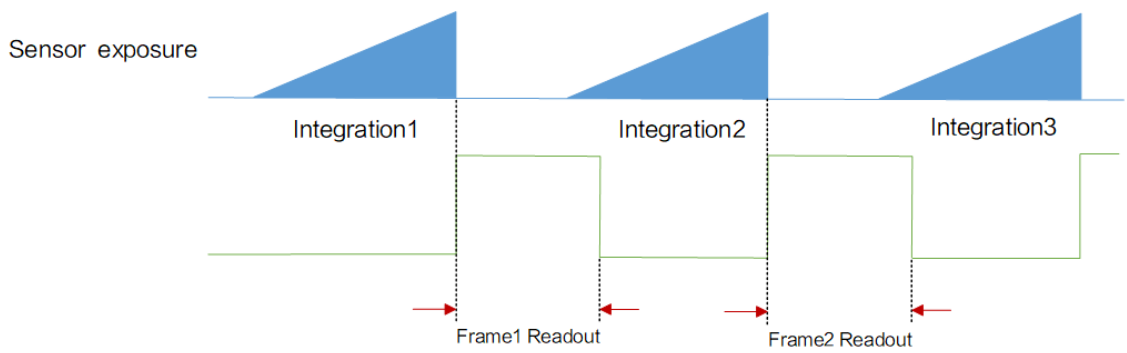
图 9-6 内触发模式
