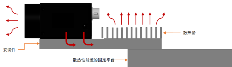
图 4-12 增加散热齿的安装件
