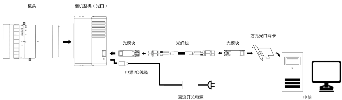
图 6-3 连接万兆光口相机
