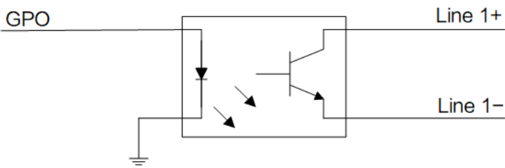
图 7-3 光耦隔离输出内部电路
