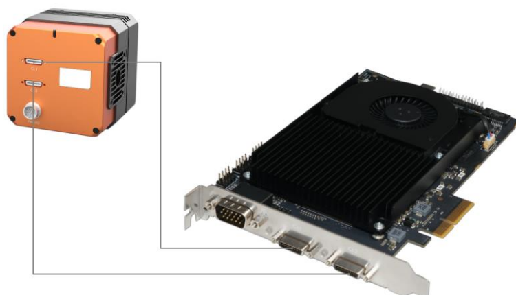
图3-3 连接单相机（2 个接口）
