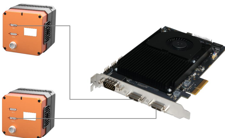
图3-4 连接双相机
