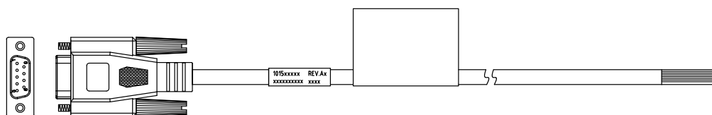
图3-7 9-Pin 转接线
