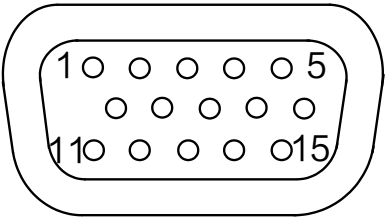
图4-1 DB15 公头
