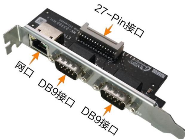
图2-5 扩展板外观
