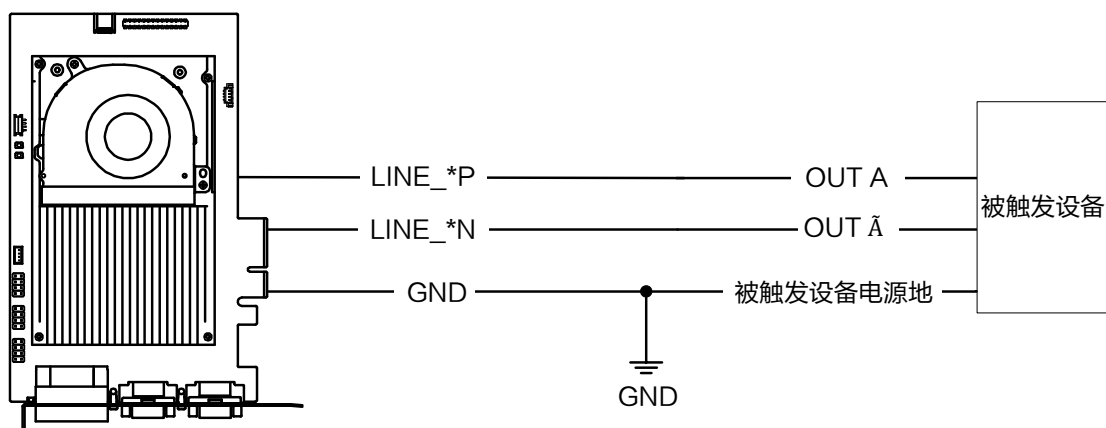
图4-11 差分输出接线
