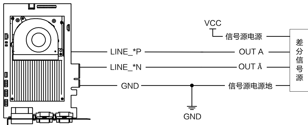
图4-6 差分输入接线
