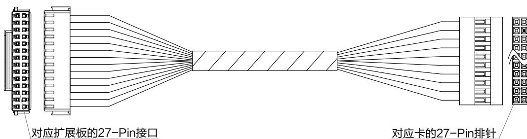
图3-5 27-Pin 转接线
