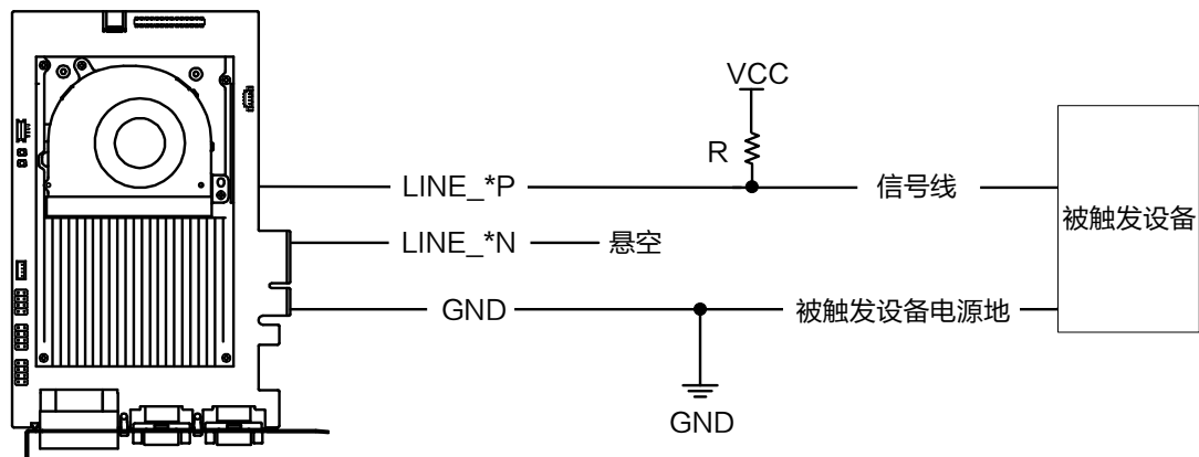
图4-12 单端输出接线（需上拉电阻）
