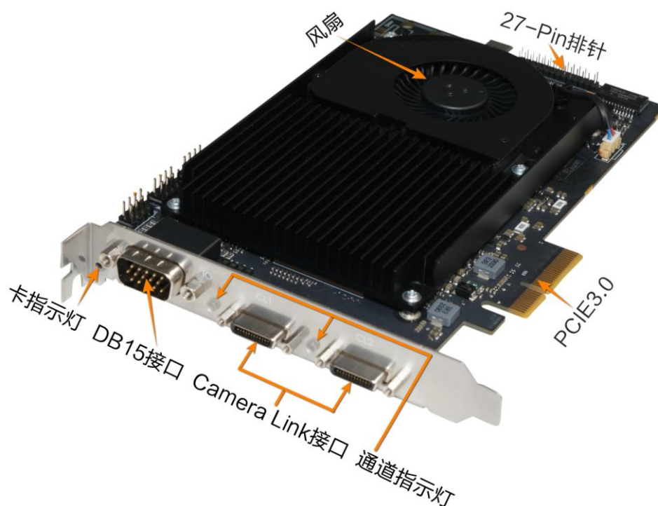
图2-1 Camera Link 视觉处理卡外观
