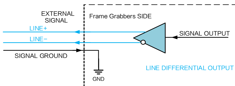
图4-5 差分输出内部电路
