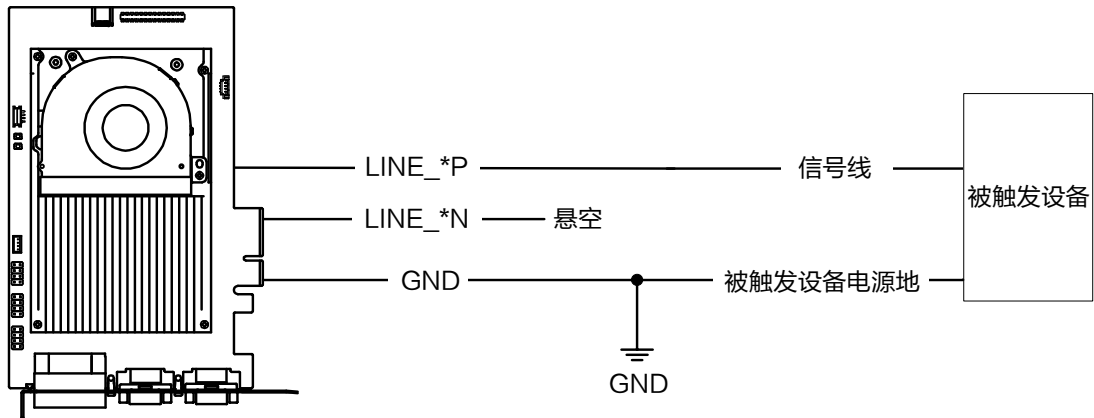
图4-13 单端输出接线（无需上拉电阻）
