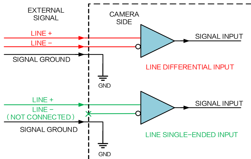
图4-4 差分输入内部电路
