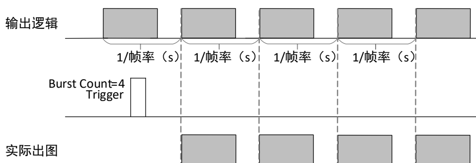
图4-13 触发出图数时序
