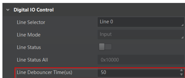
图4-19 触发防抖设置
