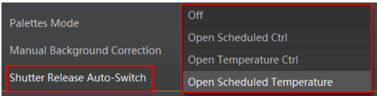
图7-6 快门控制
