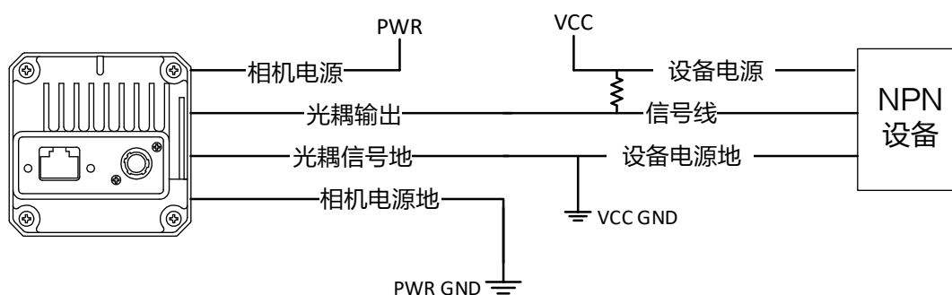
图6-12 Line 1 接 NPN 设备
