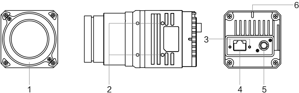
图2-1 相机外观
