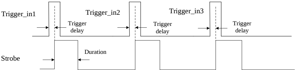
图5-7 Strobe 持续时间时序
