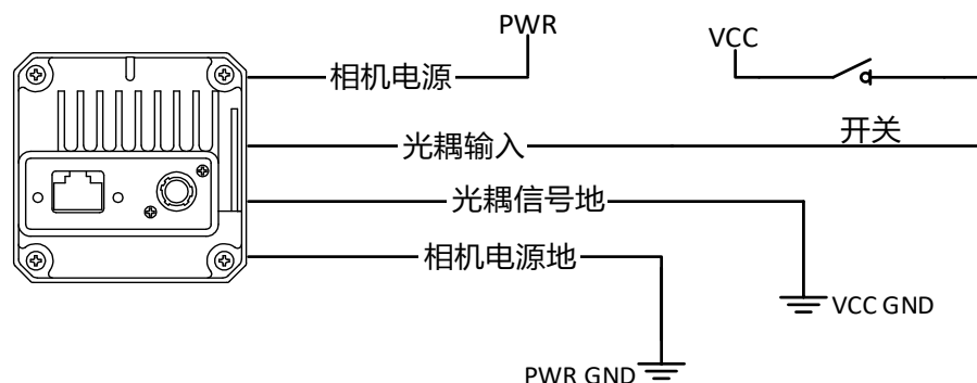
图6-10 Line 0 接开关
