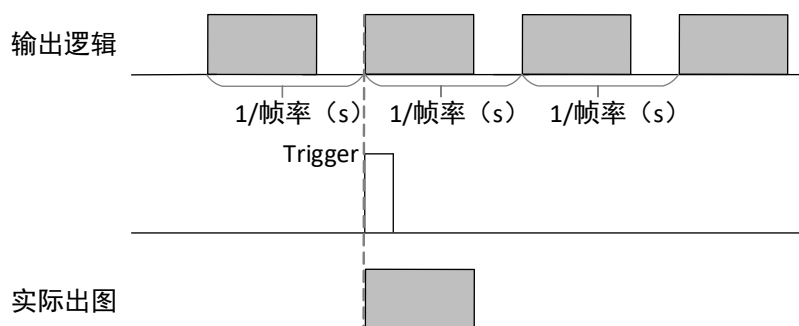
图4-3 输出当前帧图像
