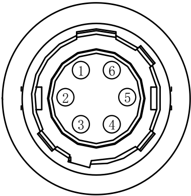
图2-3 6-pin P7 接口
