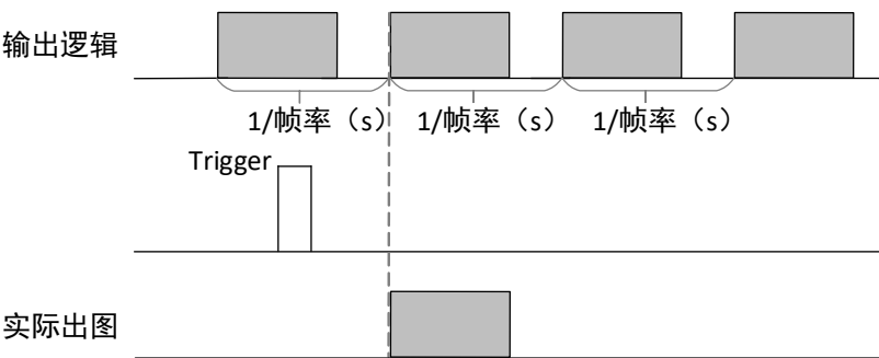
图4-4 输出下一帧图像
