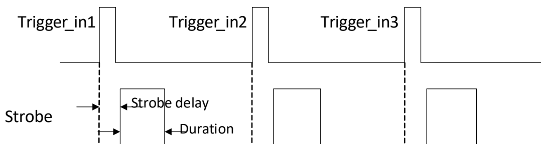
图5-9 Strobe 输出延迟时序
