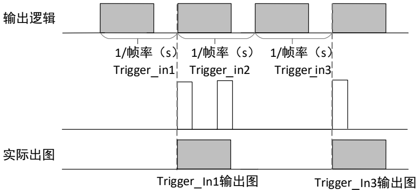
图4-16 第 2 帧被过滤时序
