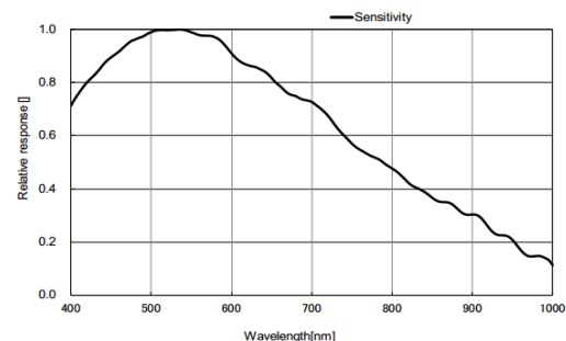
MV-CS120-10GM V5 响应曲线
