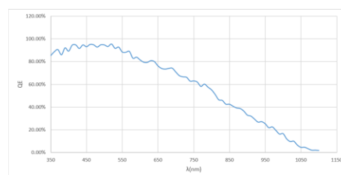
MV-CT120R-9GM01 量子效率
