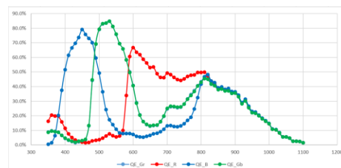
MV-CT120R-9GC01 量子效率
