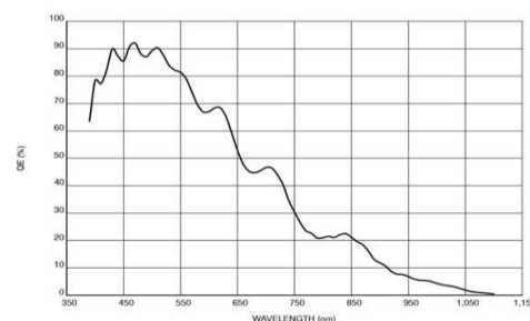
MV-CU050-30GM V2 响应曲线
