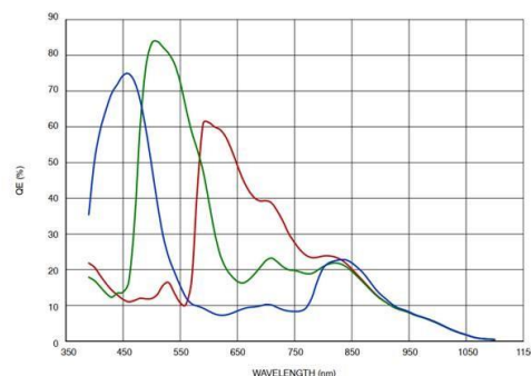
MV-CU050-30GC V2 响应曲线
