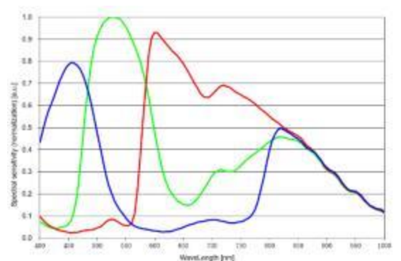
FV-4024-09RC 量子效率
