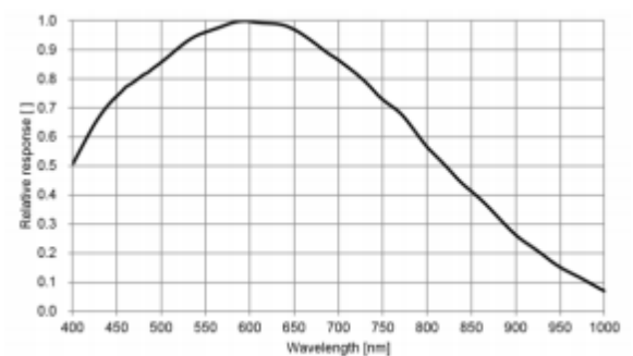
FV-4024-09RM 量子效率
