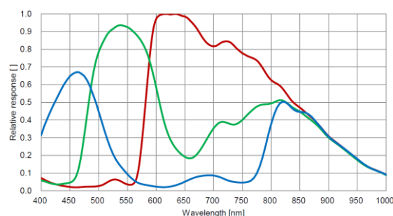
SC-HCS020-60GC 量子效率
