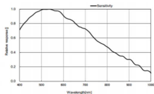
FV-4024-09RM 响应曲线
