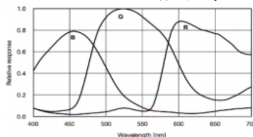
FV-4024-09RC 响应曲线
