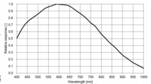
FV-5472-05RM 量子效率
