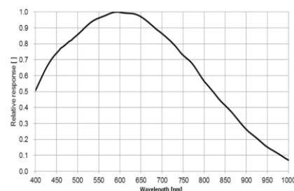
MVGL-AC245G-74UM 量子效率
