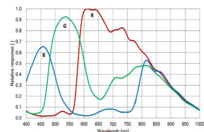
MVGL-AC245G-74UC 量子效率
