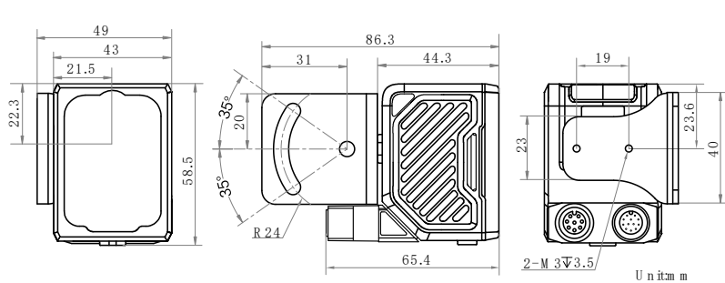
设备支架一体（直角）：
