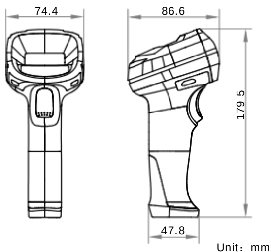
手持读码器：
