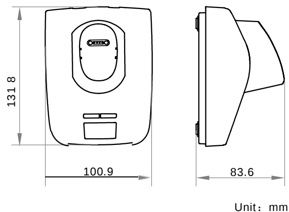
底座：
