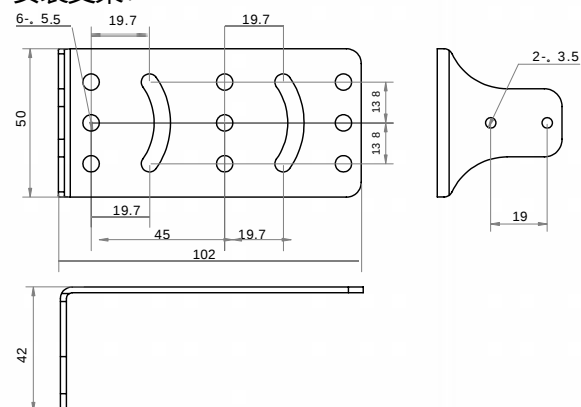
安装支架：
