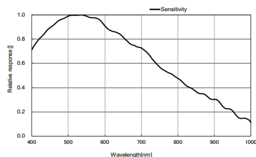
HK-YX021-9WM(NPOE)响应曲线
