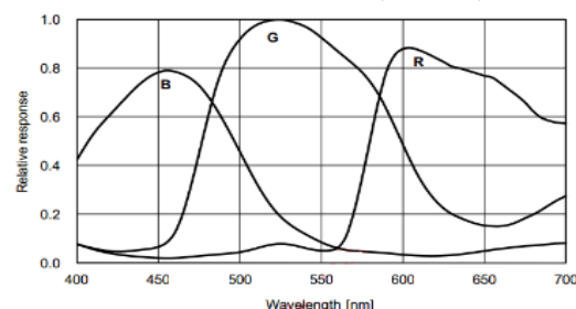
HK-YX021-9WM(NPOE)响应曲线
