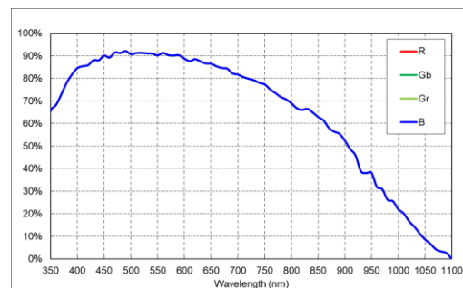
HIK-C050-MG 量子效率
