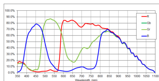
HIK-C050-CG 量子效率
