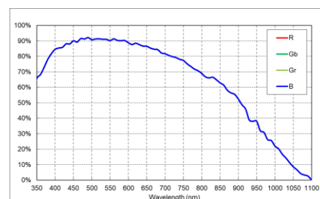
HIK-C120-MG 量子效率
