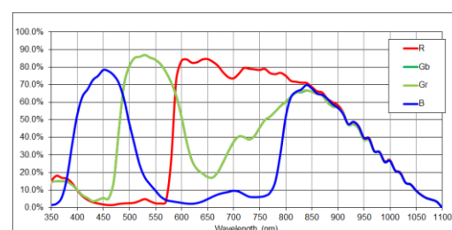
HIK-C020-CG 量子效率
