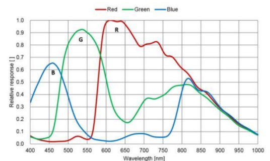
XXV-050C-XIG 量子效率
