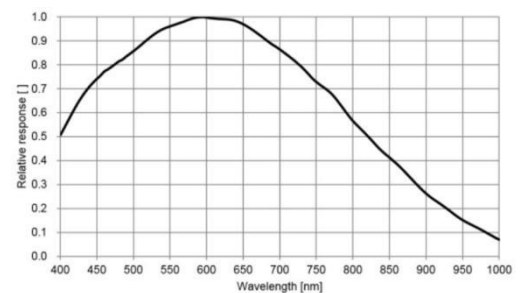
XXV-050M-XIG 量子效率
