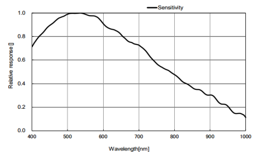
MV-DV4024-50GM 响应曲线
