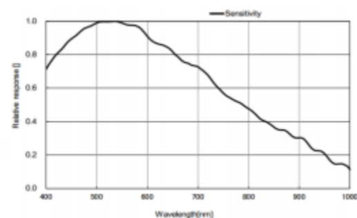
MV-XD0120-10GM 响应曲线
