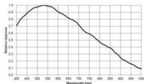
MV-XD6010GM V5 量子效率
