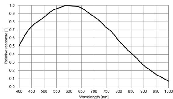
MV-SY2000-00Q-BCN 量子效率
