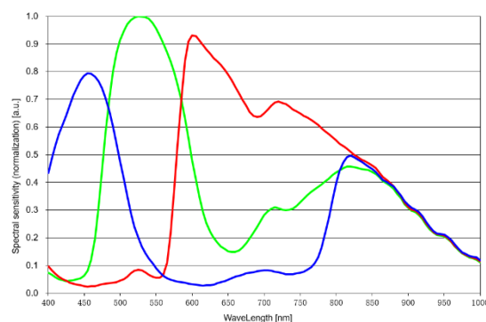
MV-SY2000-00Q-BCN 量子效率
