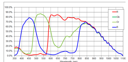
MV-HH1200-GC 量子效率
