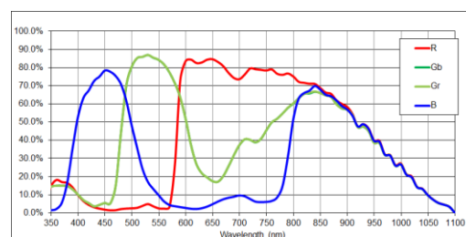
MV-HS500-GC 量子效率
