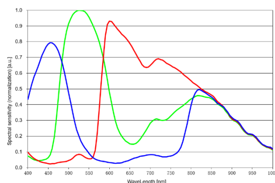
SY-2000M 量子效率
