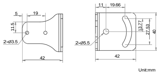
安装支架:
