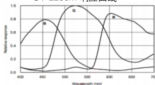
SY-1200C 响应曲线
