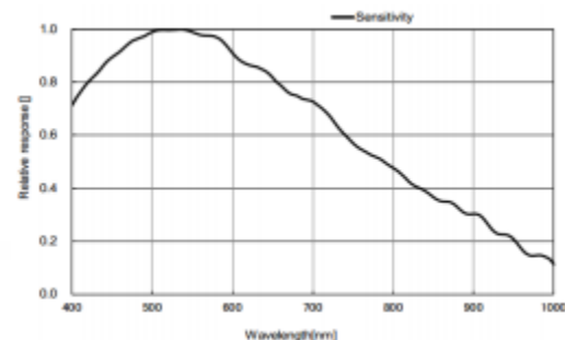
SY-1200M 响应曲线
