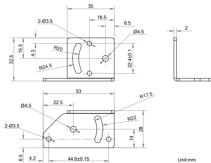
支架:
